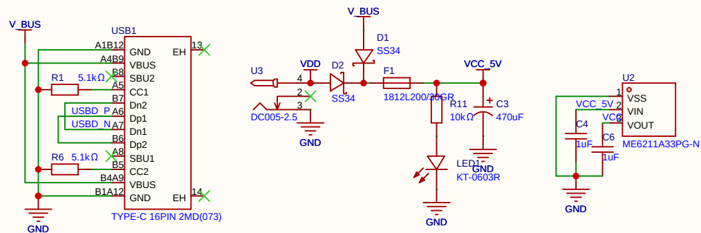
电源
