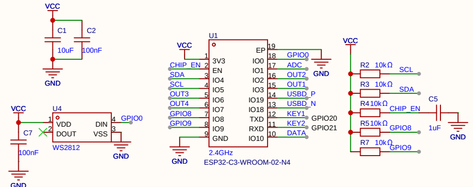
ESP32
