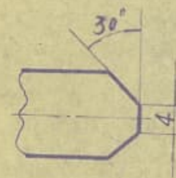
2. 焊缝坡口
