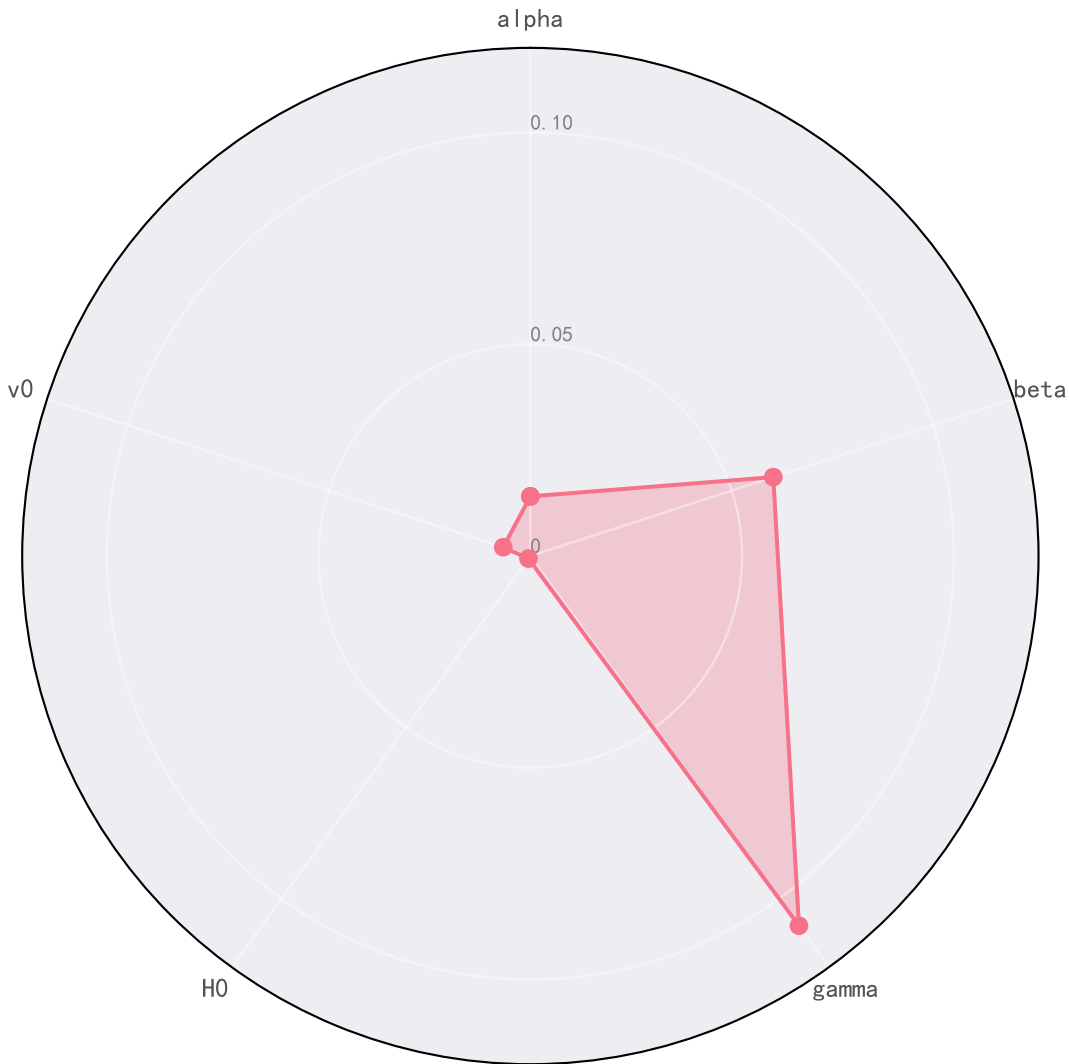
Parameter Sensitivity Radar Chart (ST Index)
