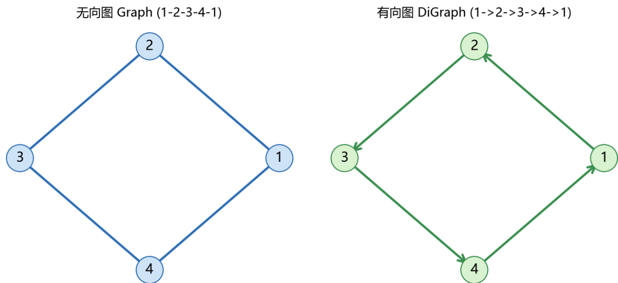
Figure 1: 无向图与有向图示例
