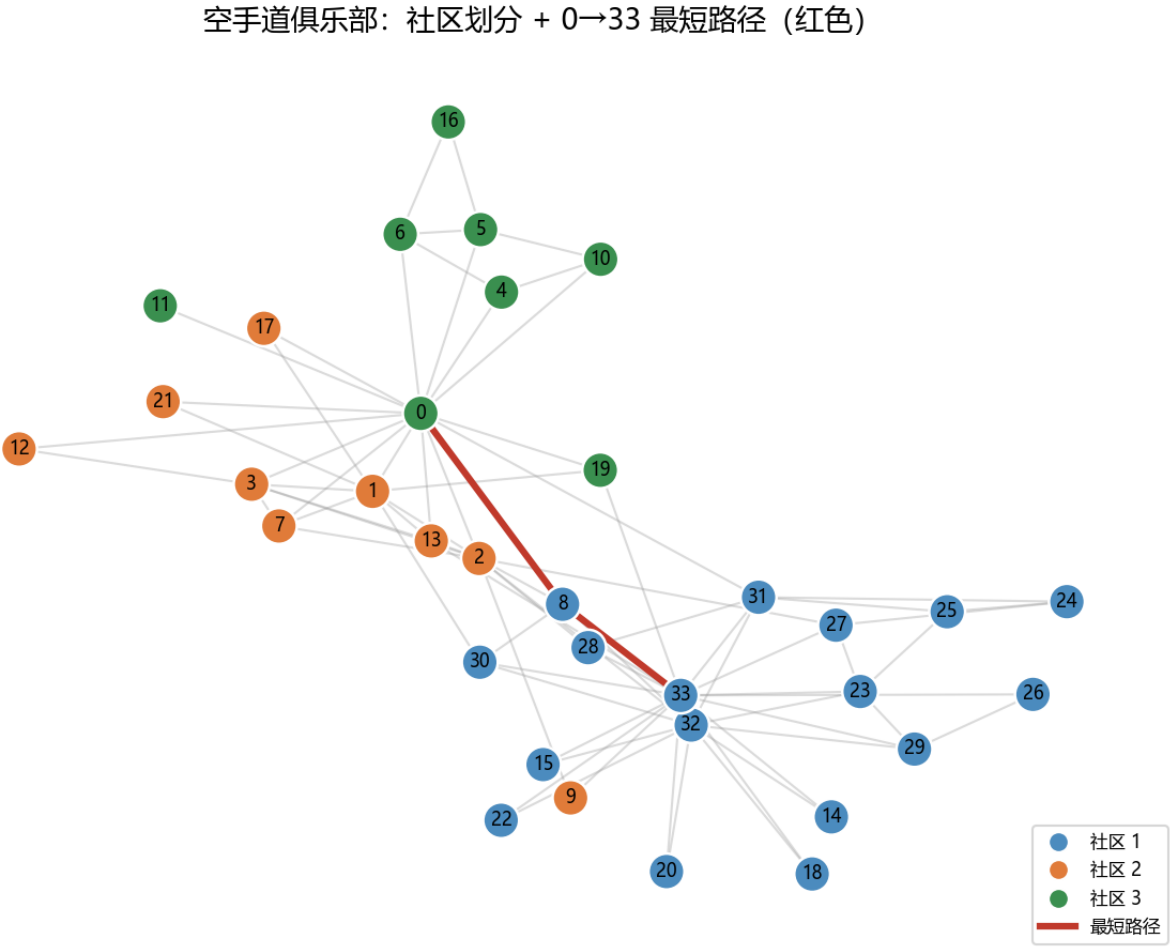
Figure 2: 空手道俱乐部 社区划分与最短路径
