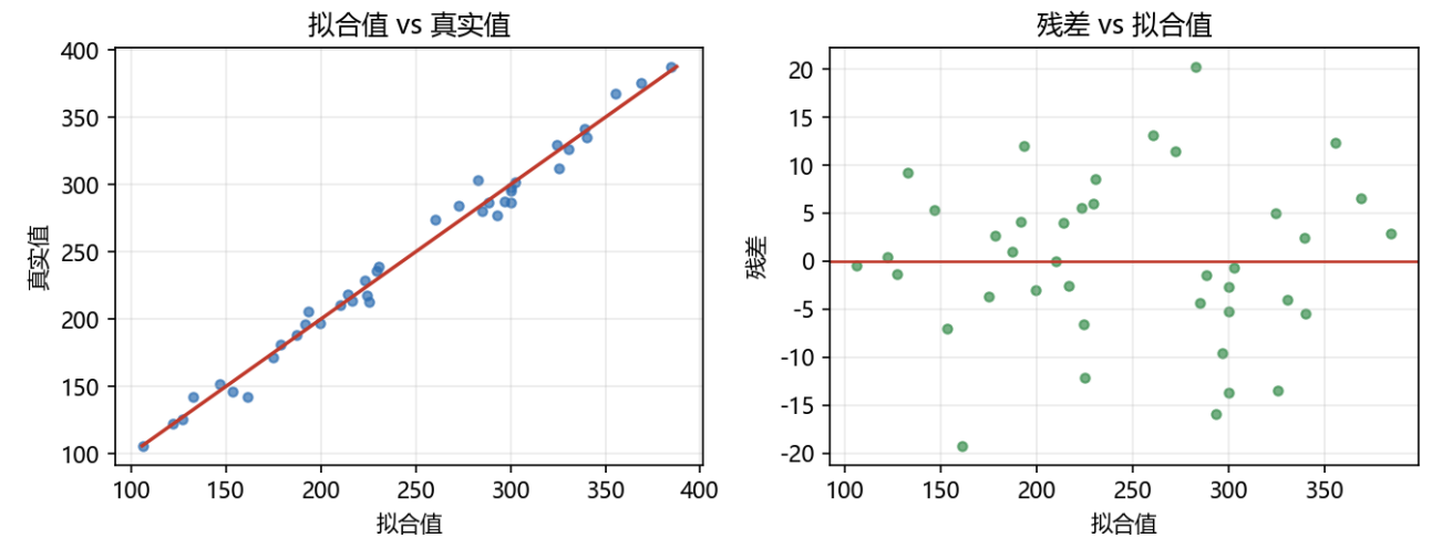
Figure 36: 拟合值 vs 真实值 与 残差图
