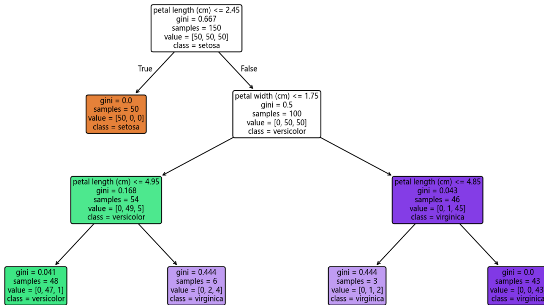
Iris 决策树 (max_depth=3)
