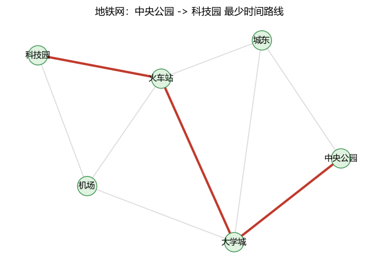
Figure 30: 地铁最少时间路线
