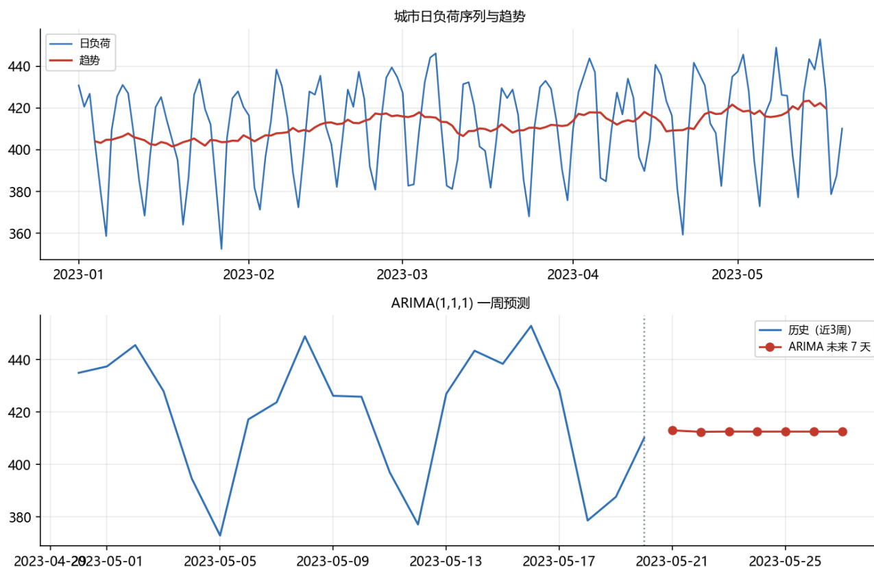
Figure 42: 时间序列：序列趋势与 ARIMA 一周预测
