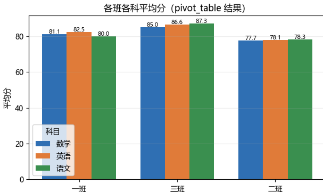
Figure 16: 各班各科平均分
