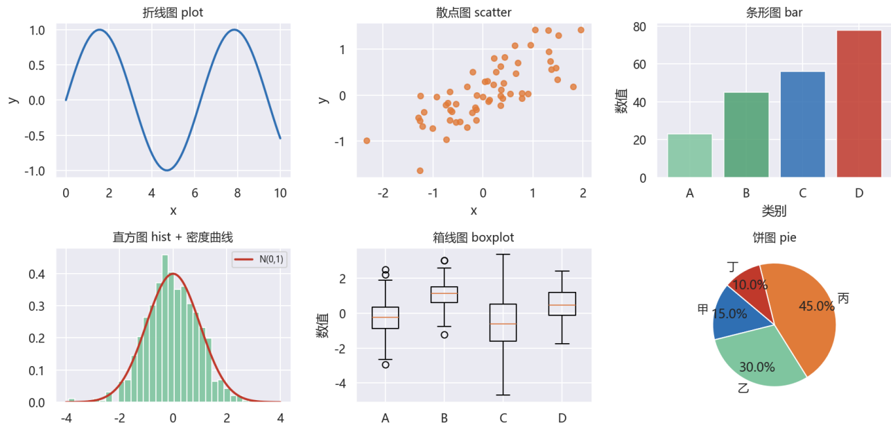
Figure 19: 基础图表一览
