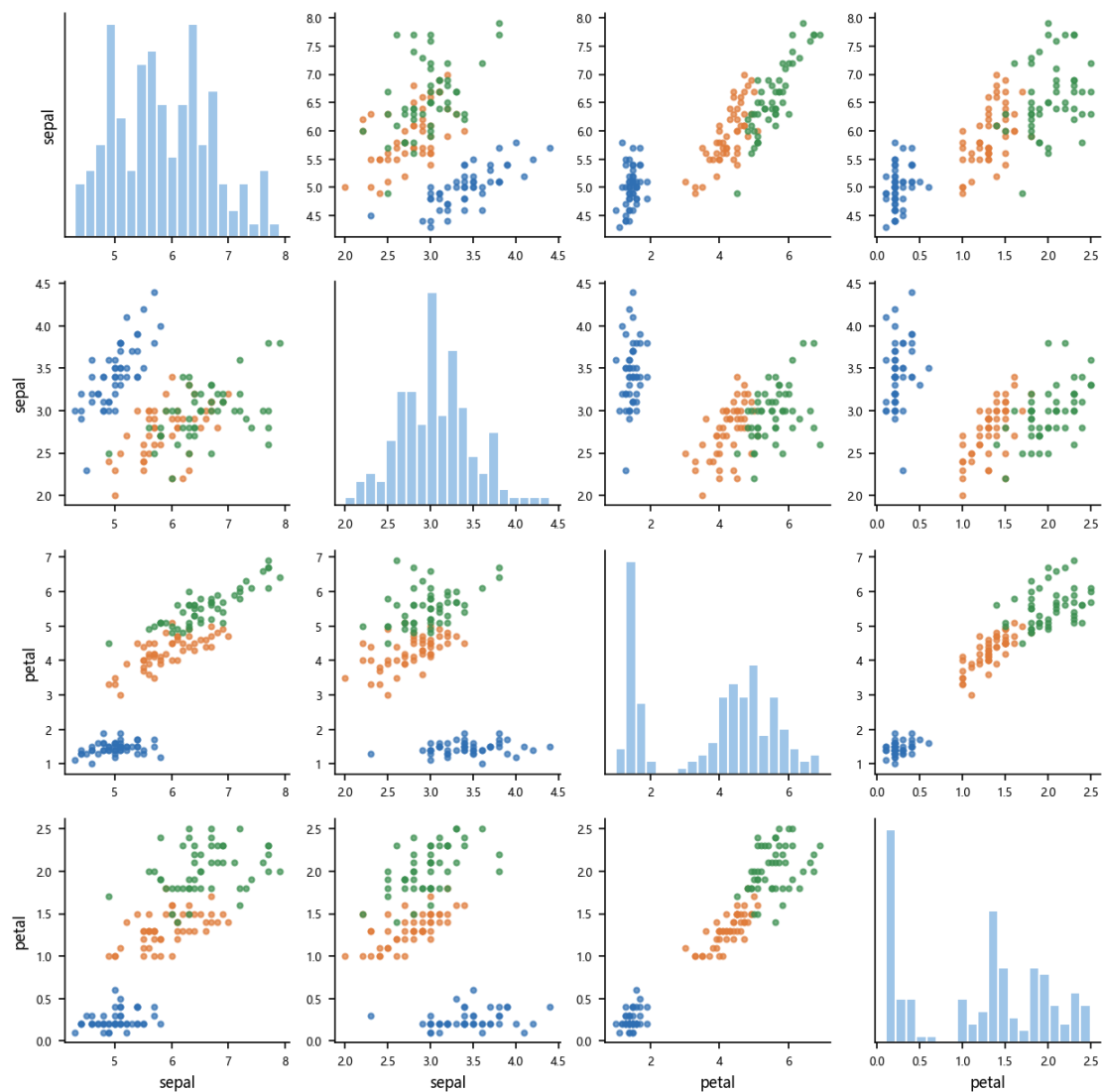
Figure 43: Iris 特征两两分布
