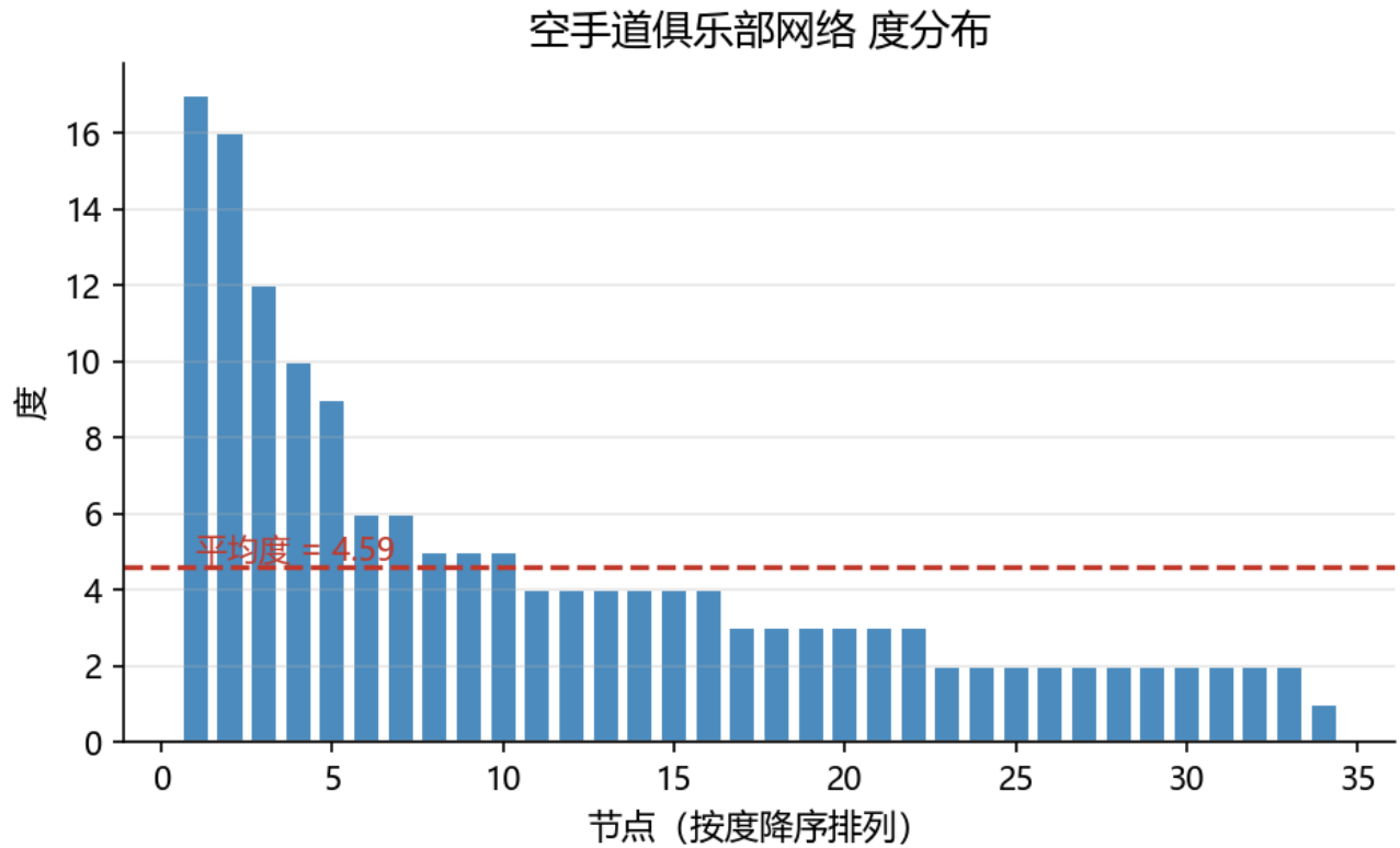
Figure 31: 空手道俱乐部 度分布
