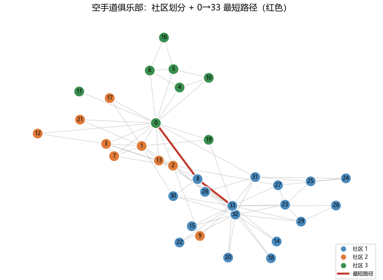
Figure 32: 空手道俱乐部 社区划分与最短路径
