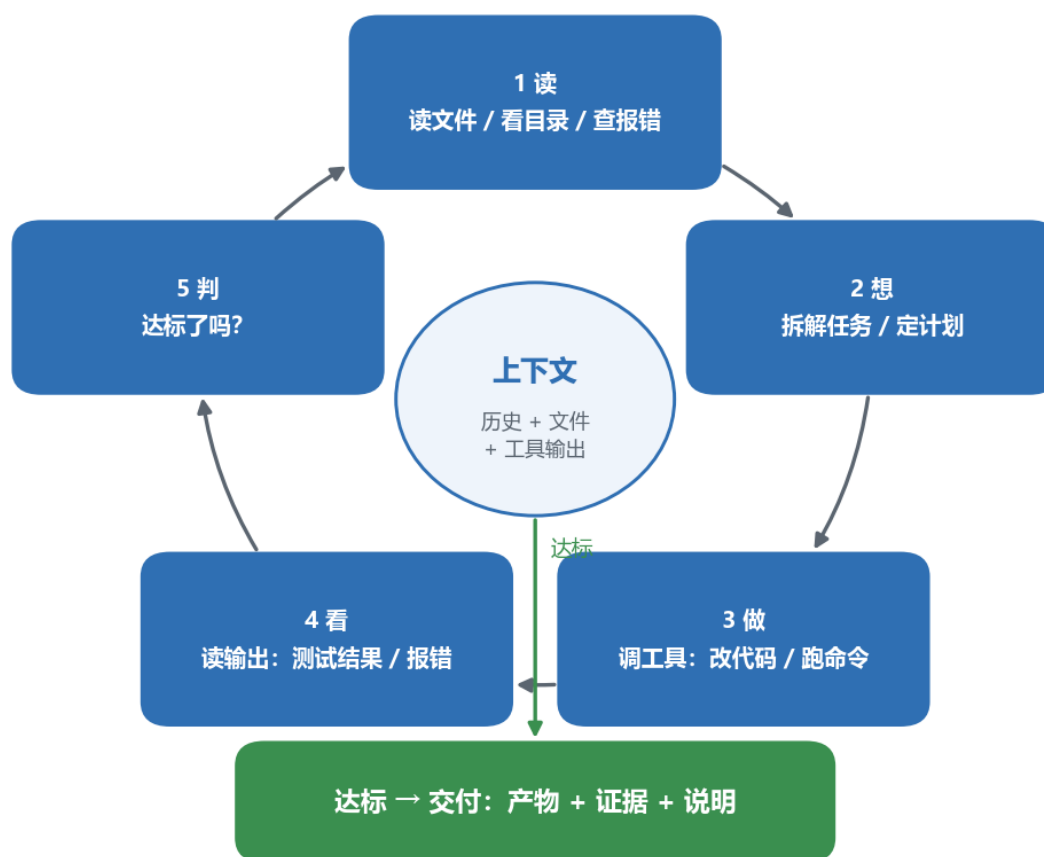
Figure 52: 一次 Agent 循环
