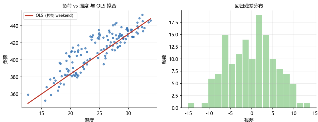
Figure 41: 回归诊断：负荷-温度散点与残差分布
