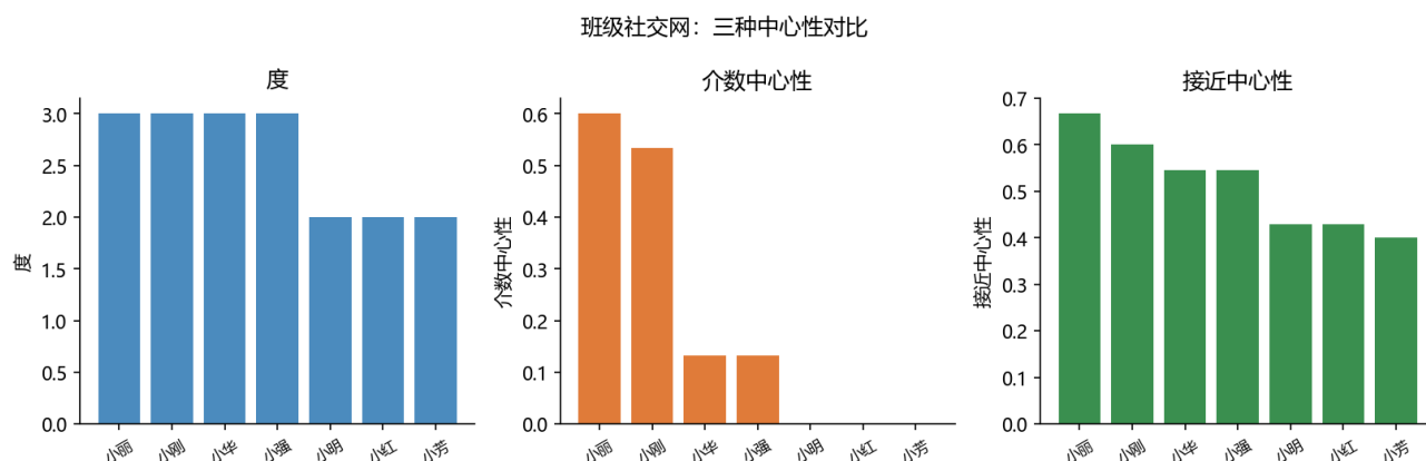
Figure 29: 三种中心性对比
