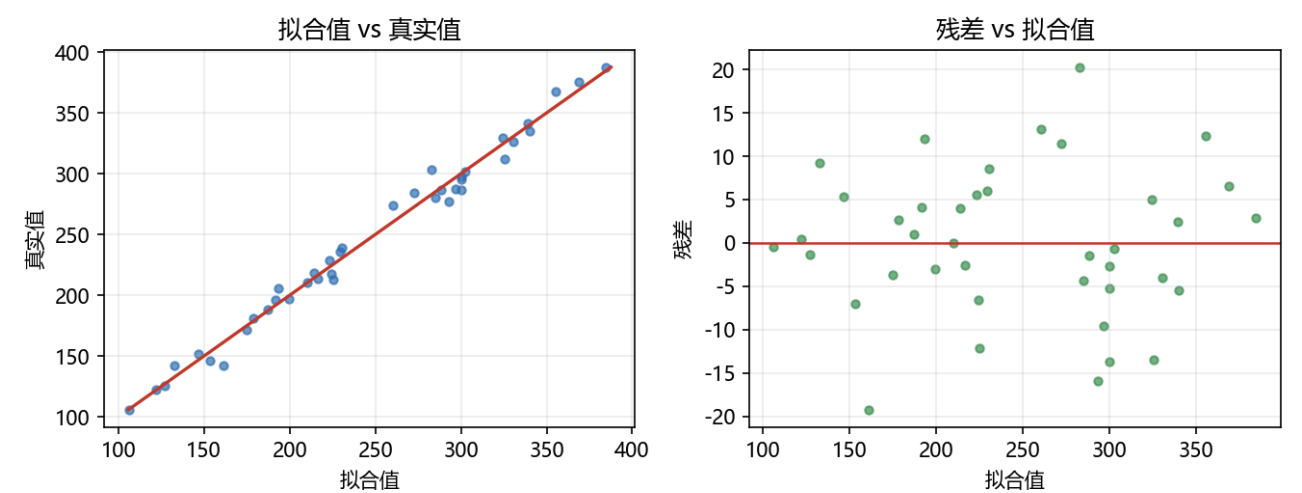
Figure 36: 拟合值 vs 真实值 与 残差图
