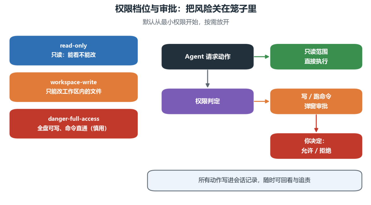
Figure 54: 权限档位与审批
