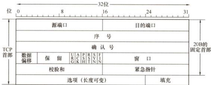
图 2 TCP 段头结构
