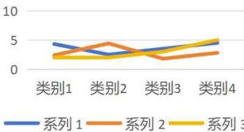
do均值及方差
