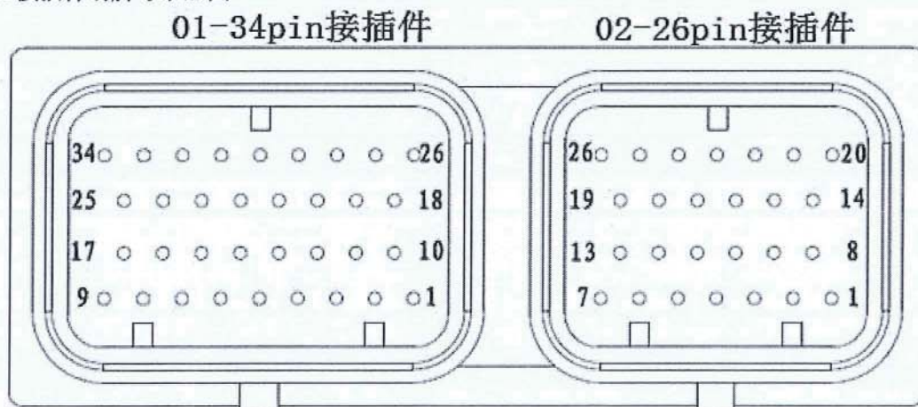
60pin 接插件引脚号示意图
