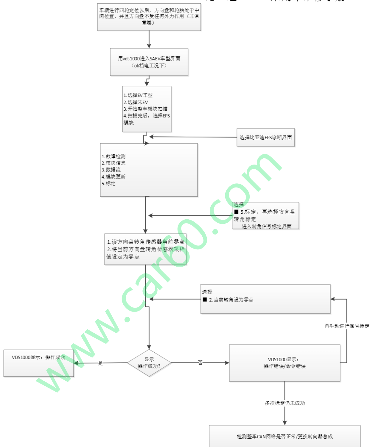
图3-1、转角信号标定流程
