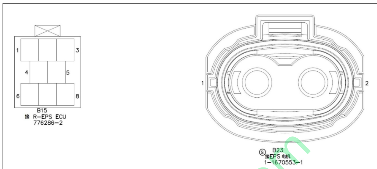
图 2-2 R-EPS 线束端引脚定义（测试端视图）
