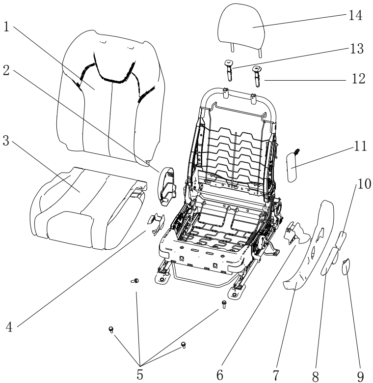
图 6.2 手动调节主驾驶座椅
