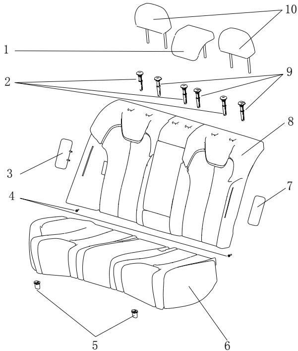
图 6.5 高配后排座椅
