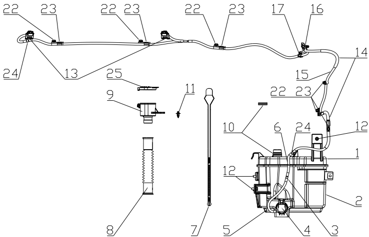
图 6.13 洗涤系统总成
