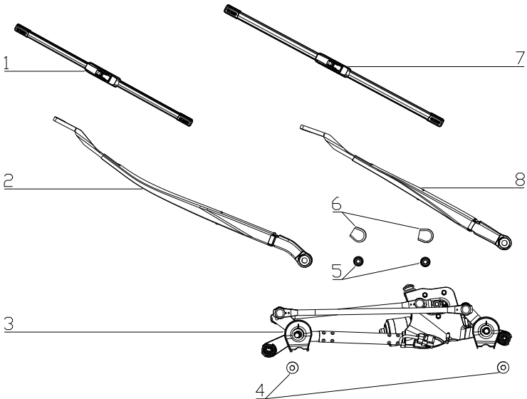
图 6.14 雨刮系统总成
