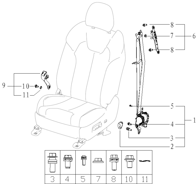
图 6.8 左前安全带总成
