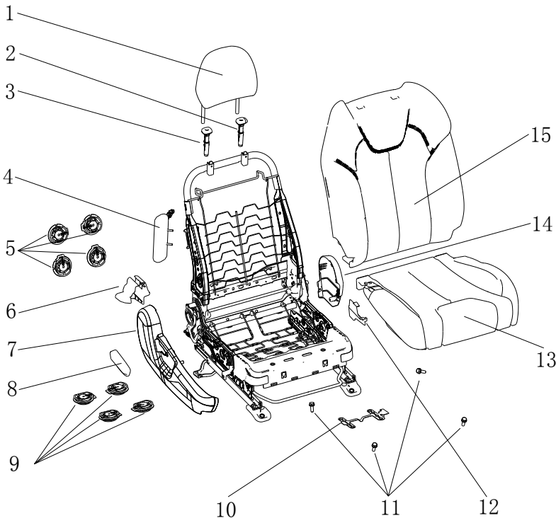
图 6.3 手动调节副驾驶座椅（高配）
