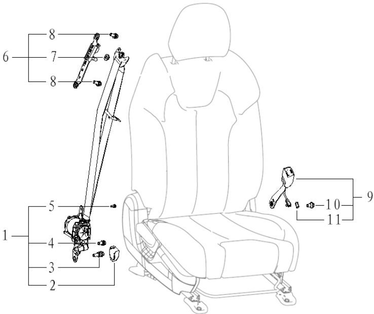
图 6.9 右前安全带总成
