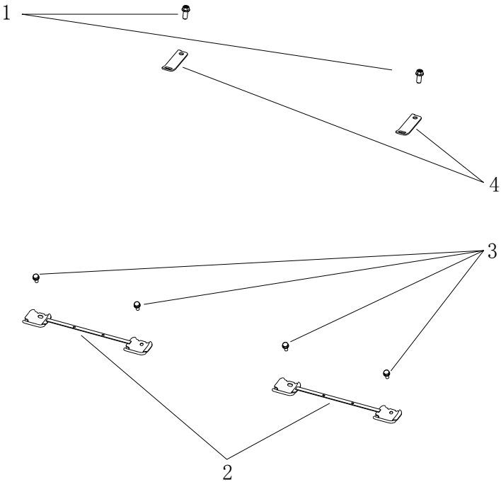
图 6.7 儿童座椅固定点
