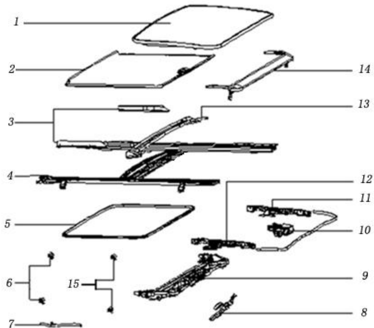
图 6.17 天窗总成
