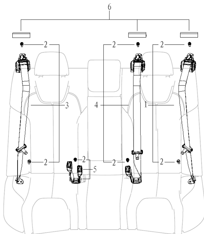
图 6.10 后排安全带总成
