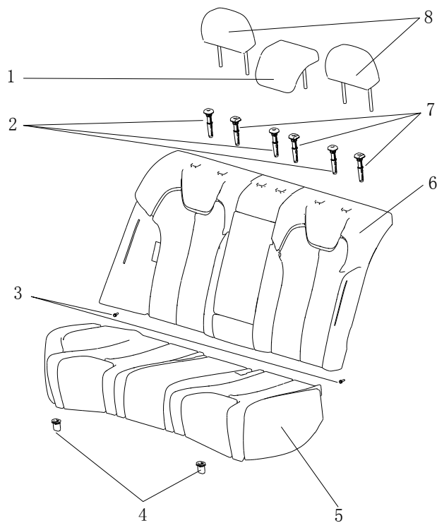
图 6.6 低配后排座椅
