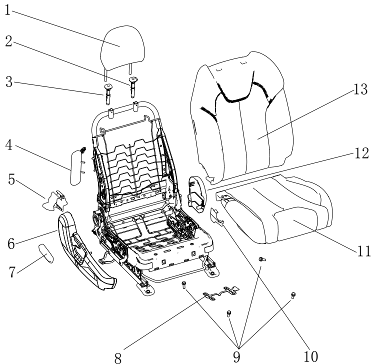
图 6.4 手动调节副驾驶座椅（低配）
