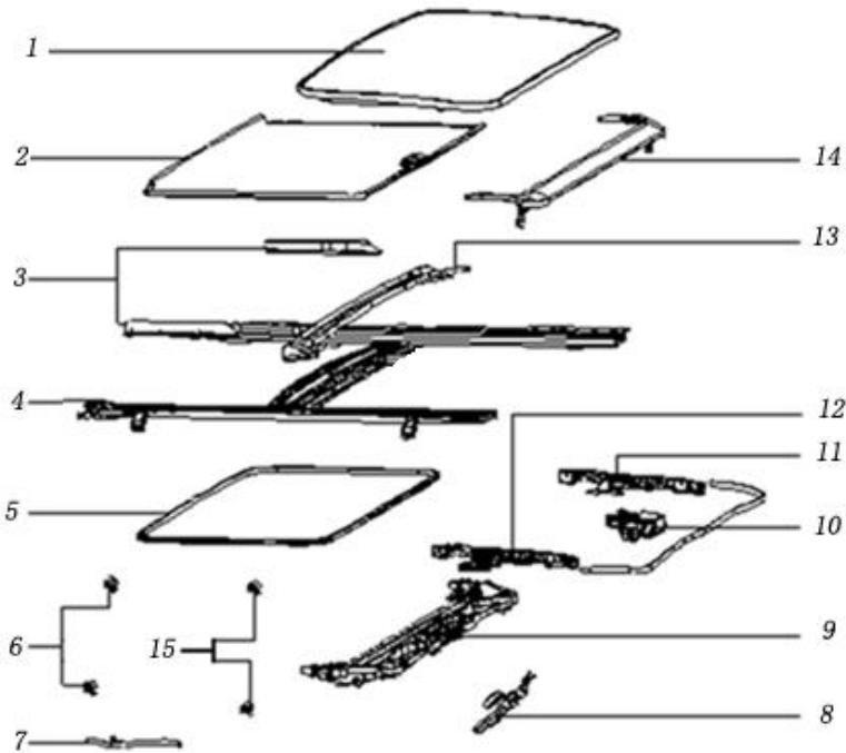
图 6.17 天窗总成
