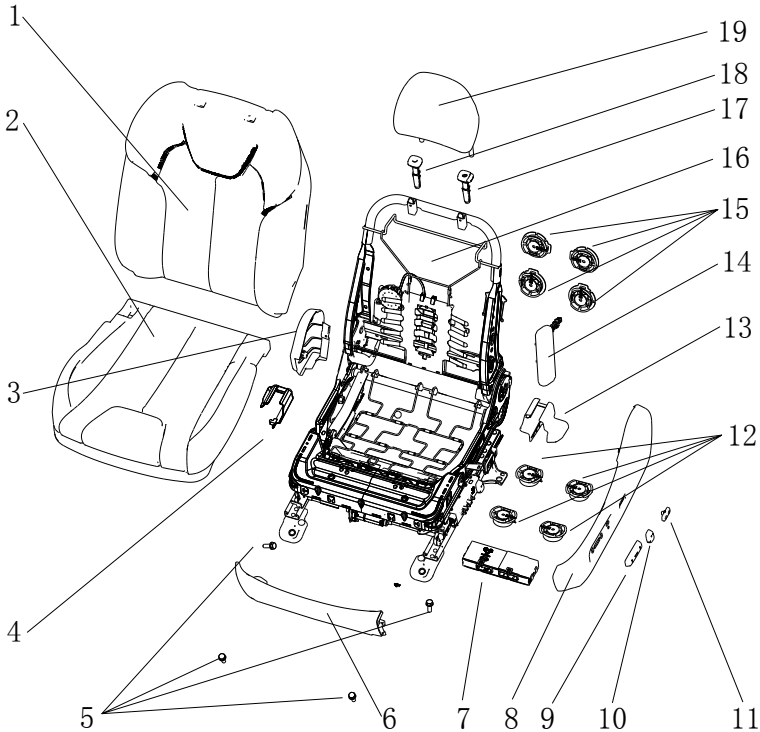
图 6.1 电动调节主驾驶座椅
