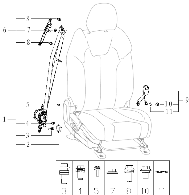
图 6.9 右前安全带总成
