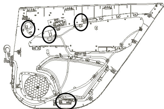
图1.9.22 线束拆卸
