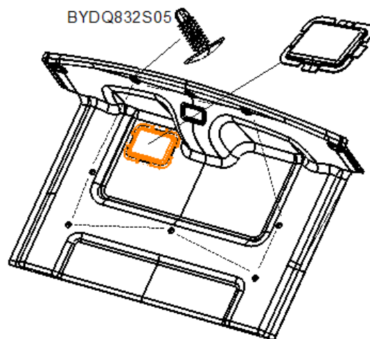
图 1.15.3 行李箱检修口盖板安装结构图
