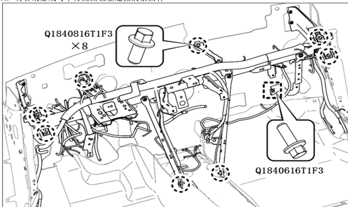
图 1.5.24 管梁总成
