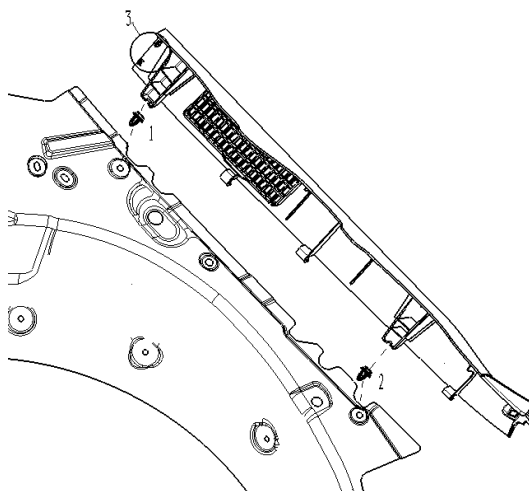
图 1.7.10 C 柱下护板拆卸
