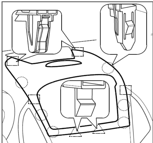
图 1.5.20 DVD 屏罩总成装配状态
