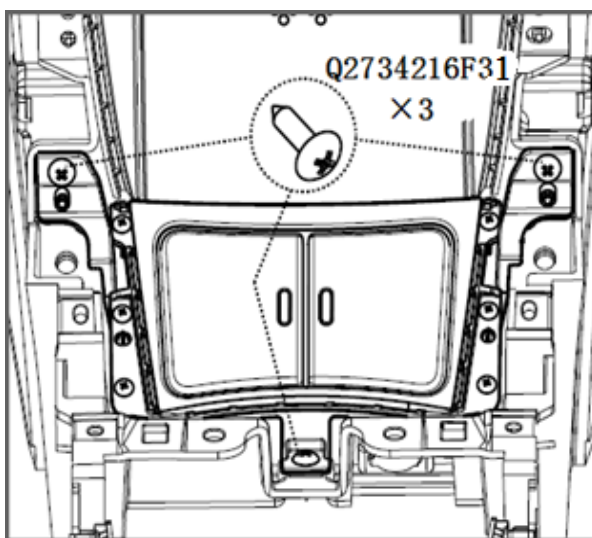
图 1.6.9 前烟灰盒总成的拆卸
