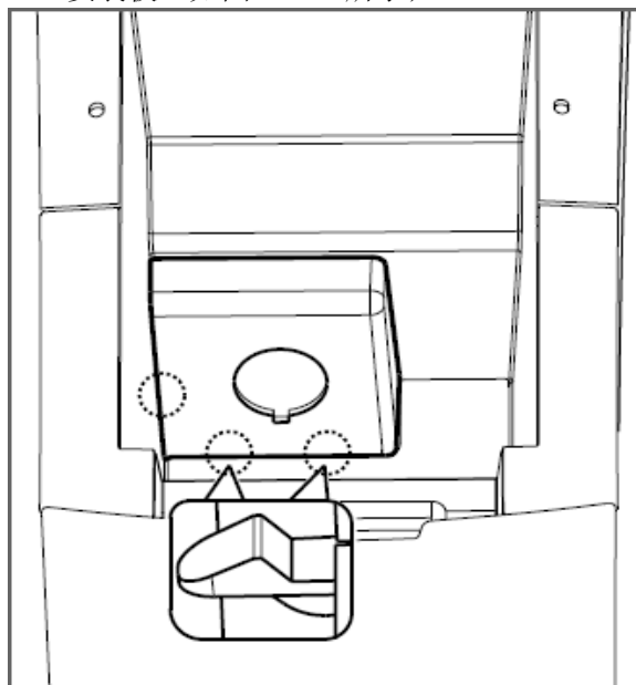
图 1.6.11 备用电源安装板的拆卸 a
