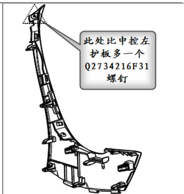
图 1.5.18 中控右护板
