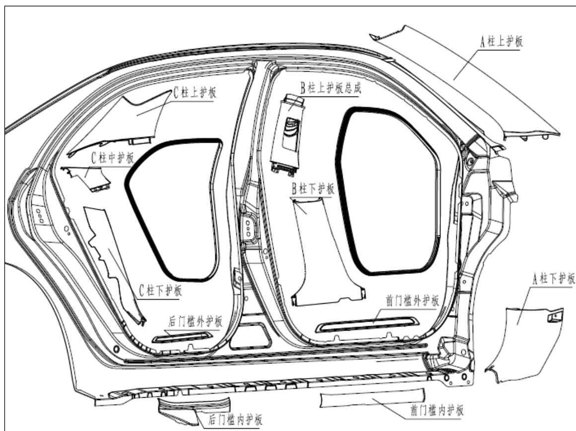
图 1.7.1 侧围系统
