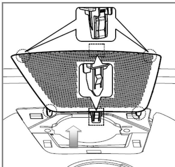
图 1.5.20 中央扬声器罩装配状态
