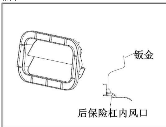
图 1.2.4 保险杠内风口的拆卸
