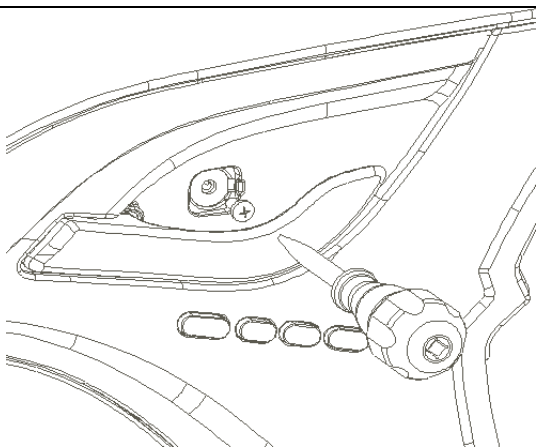
图1.9.6 内扣手螺钉
