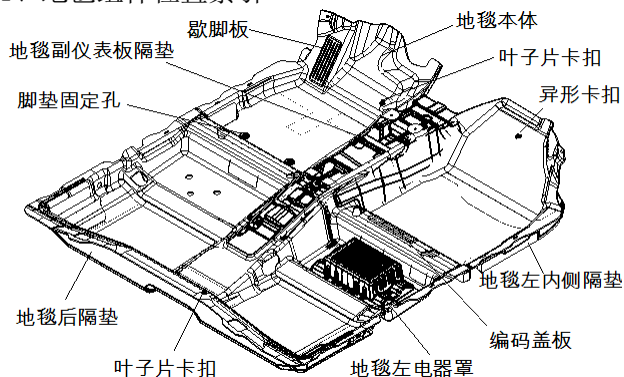
图 1.13.1 地毯总成结构示意图
