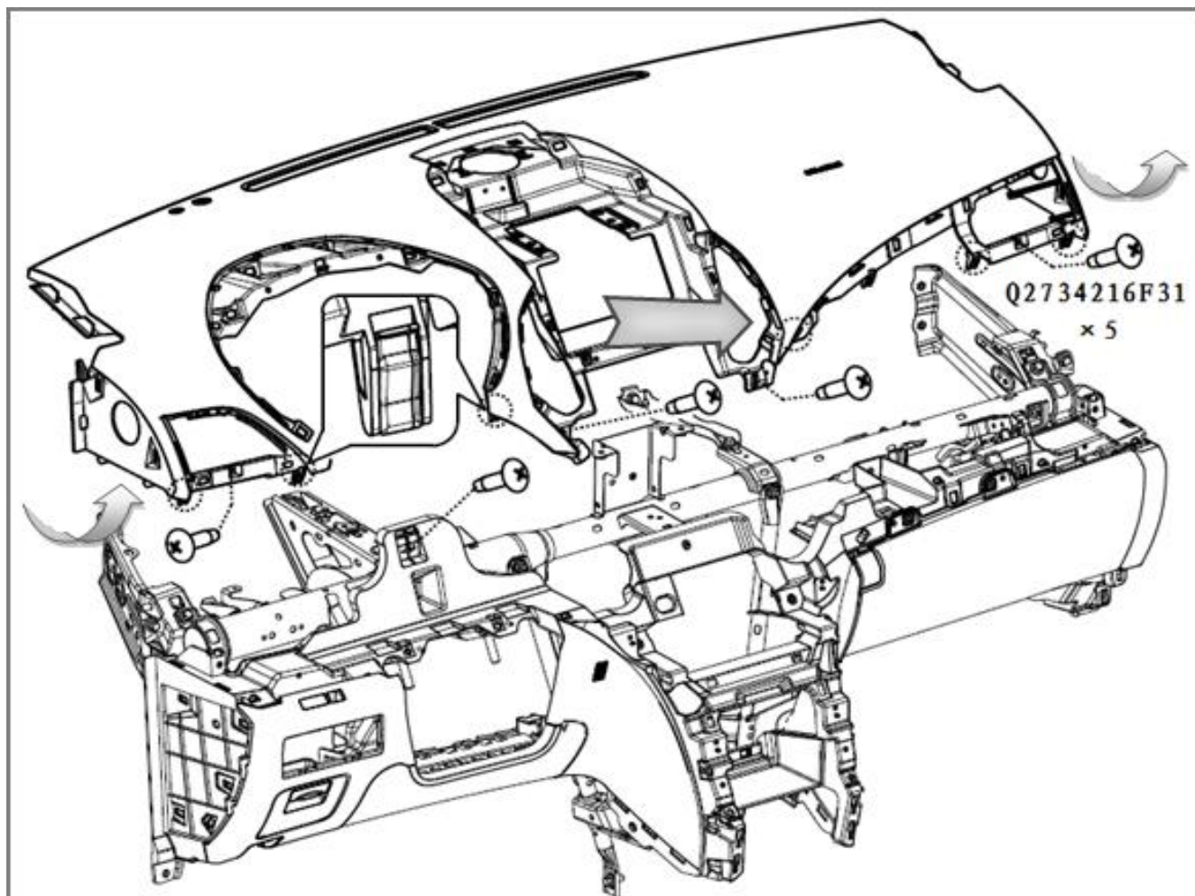
图 1.5.22 仪表板上本体拆卸示意图
