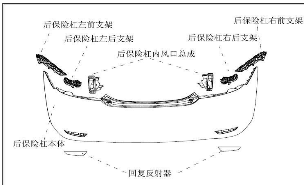
图1.2.1后保险杠系统组件
