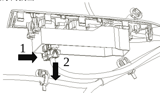
图1.9.4 窗控面板接插件
