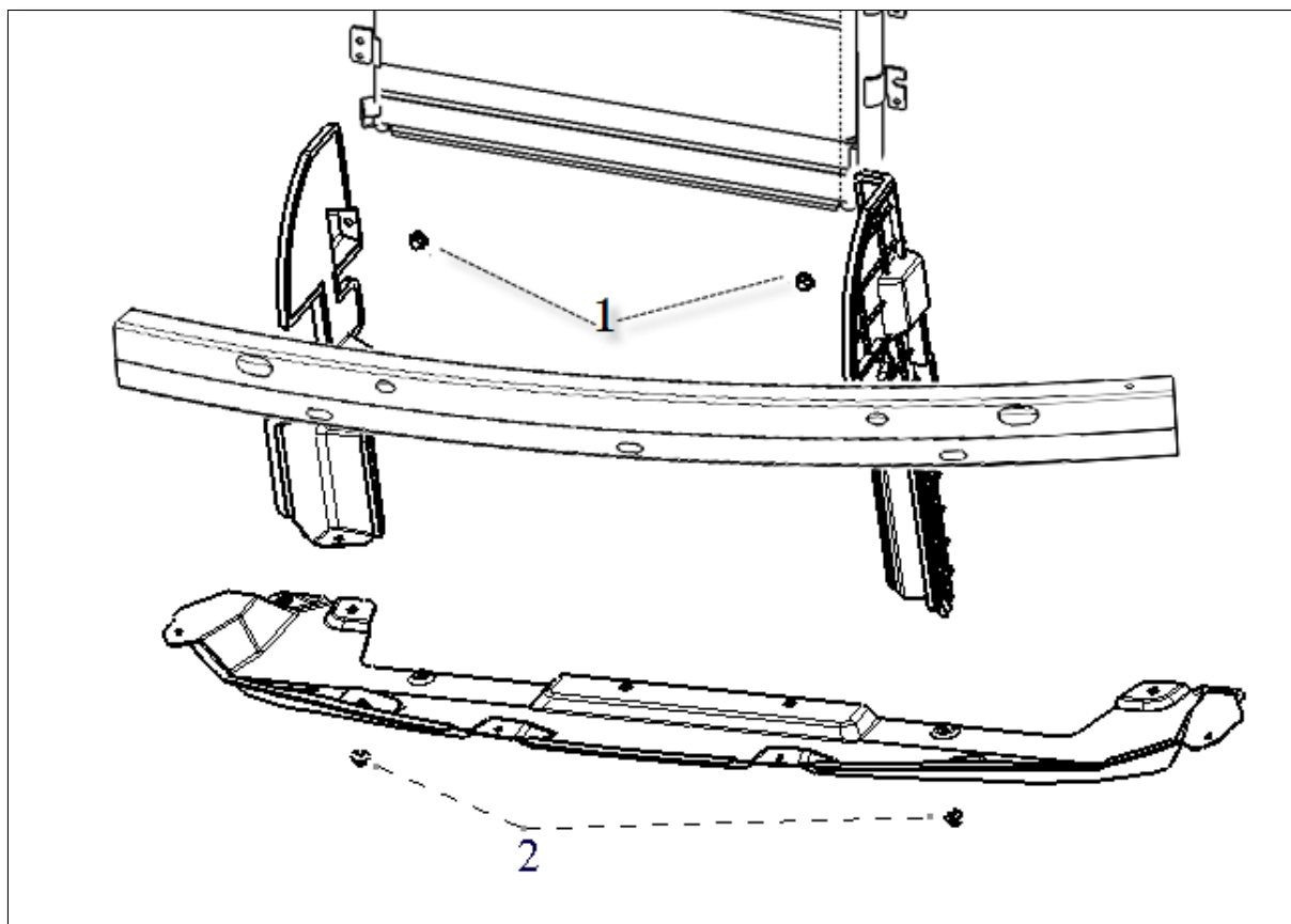
图 1.3.4 导流板的拆卸/安装
