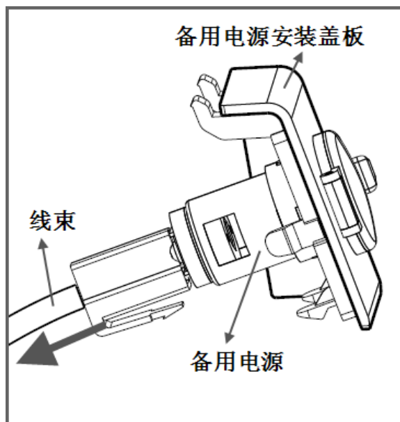
图 1.6.12 备用电源安装板的拆卸 b
