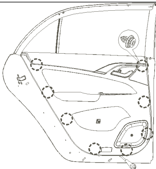
图1.9.18 门板拆卸
