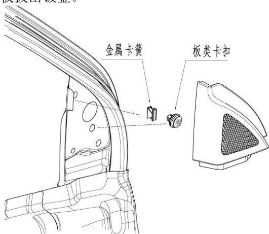
图1.9.11 角护板拆卸
