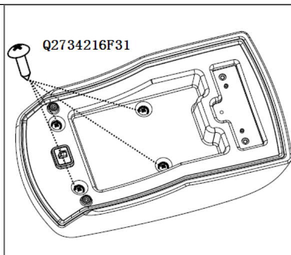
图 1.6.21 副仪表板扶手组件的分拆 2
