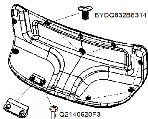
图 1. 15.4 行李箱盖护面 安装结构图
