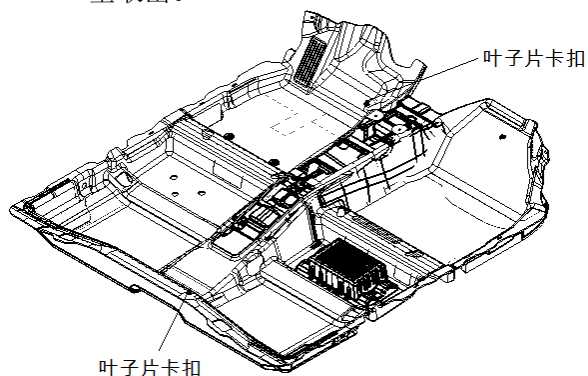
图 1.13.2 地毯安装结构示意图
