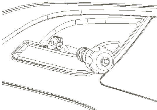
图1.9.17 内扣手螺钉
