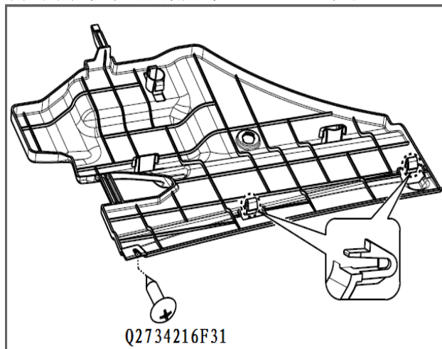
图 1.5.3 仪表板右下隔音板组件
