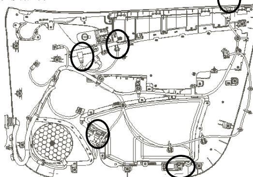
图1.9.10 线束拆卸
