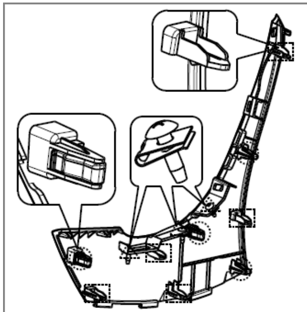
图 1.5.17 中控左护板
