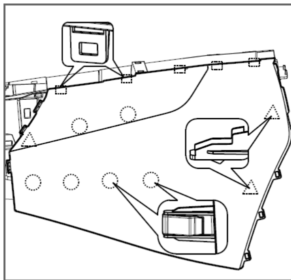
图 1.6.18 副仪表板左、右护板总成的拆卸
