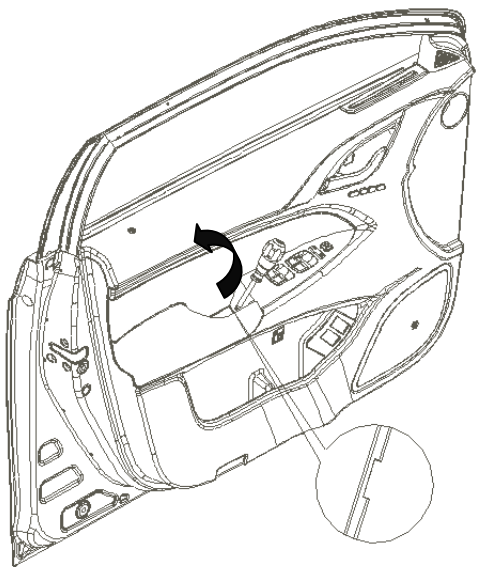
图1.9.1 内拉手盖板
