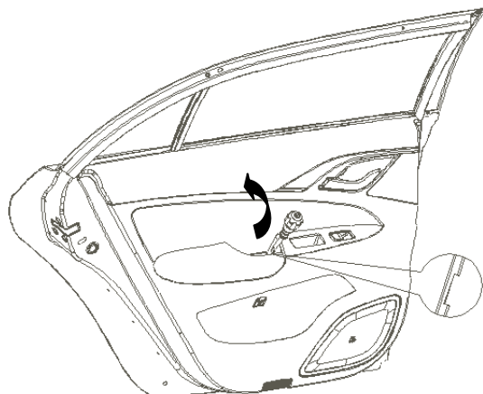
图1.9.12 内拉手盖板
