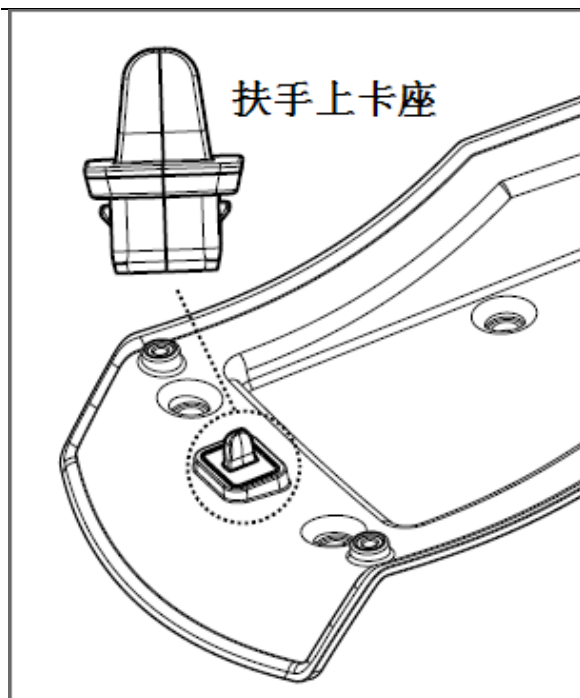
图 1.6.23 副仪表板扶手上卡座的拆卸
