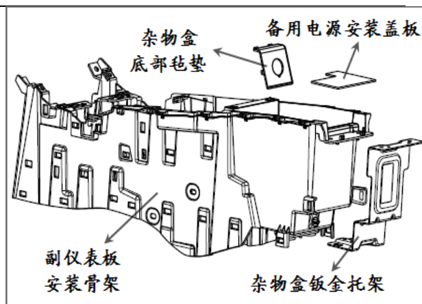
图 1.6.3 副仪表板本体总成 2
