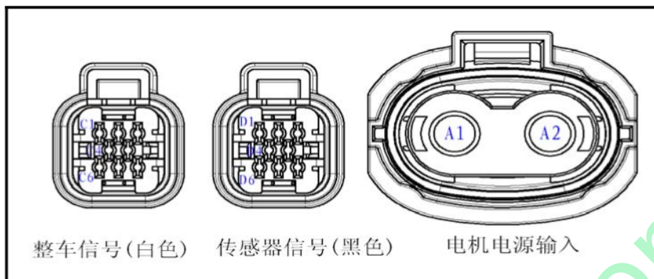
图 3 R-EPS 线束端引脚定义（测试端视图）
