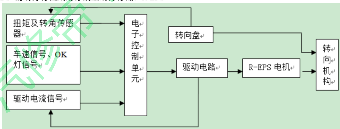
图 1 R-EPS 系统工作原理
