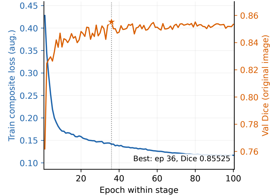
A: CNN DONE 100/100
