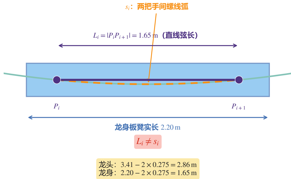
(b) 局部放大：固定的是直线弦长，而非螺线弧长
