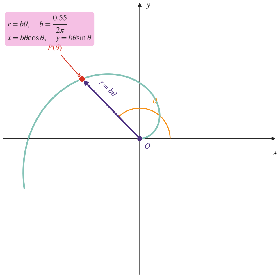
(b) 极坐标参数的局部定义
