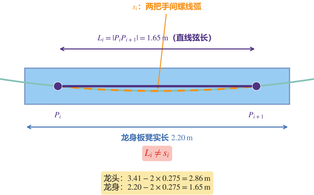
(b) 局部放大: 固定的是直线弦长, 而非螺线弧长
