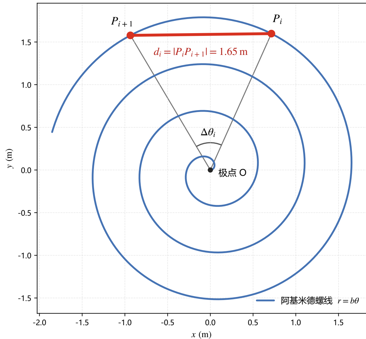
图2 相邻把手几何约束示意图
