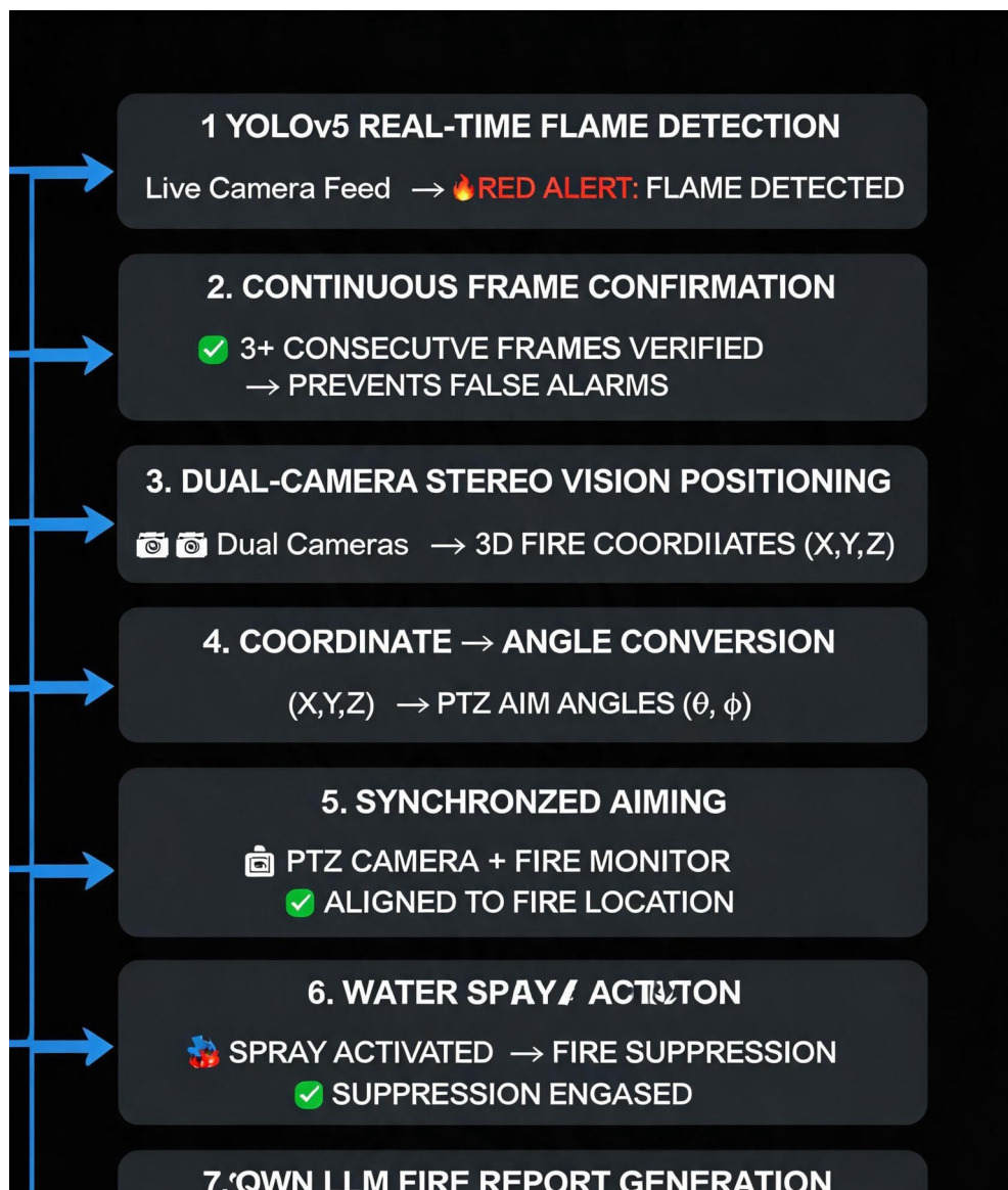
图 4-4 火焰检测与联动流程图
