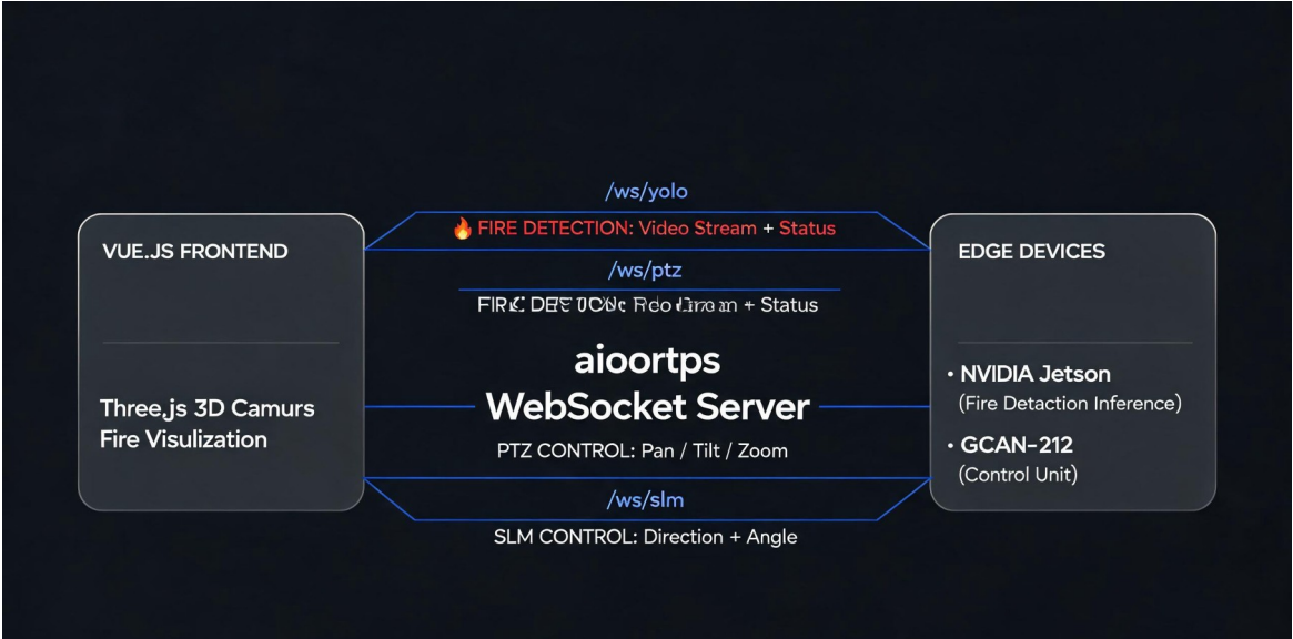
图 4-3 三路 WebSocket 连接架构图
