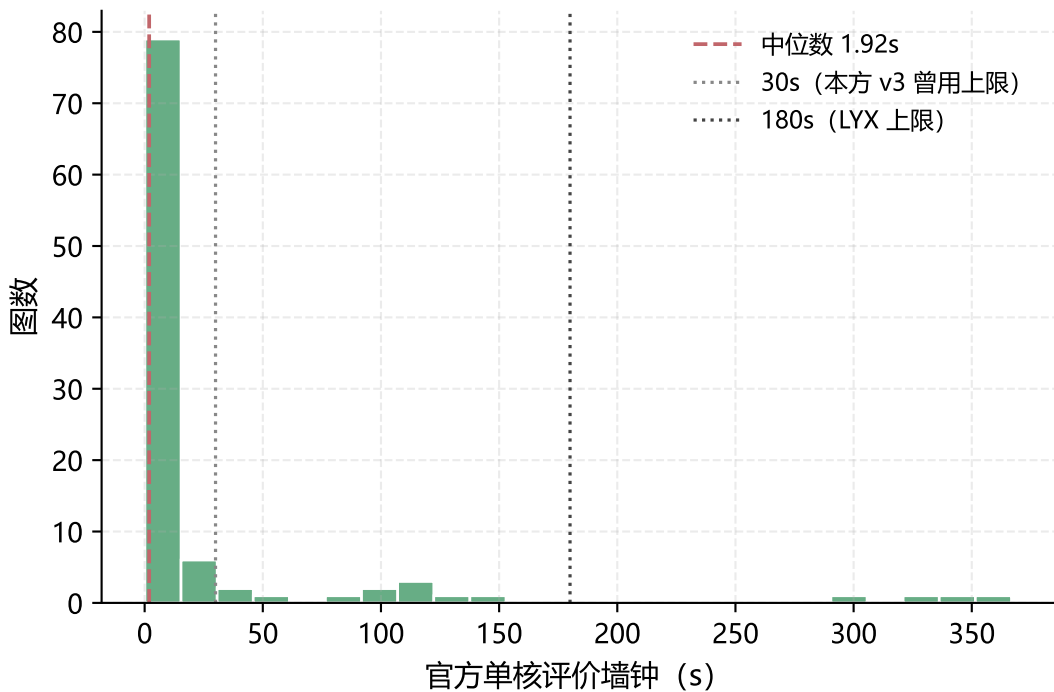
官方单核分母逐例墙钟分布 (n=100/100, Batch C)
