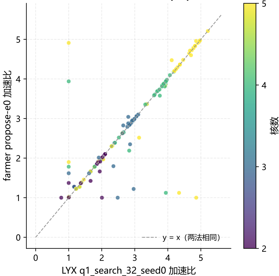
P1 双算法同格并列 (n=180; 对角线上方=propose 更优 64 格)
