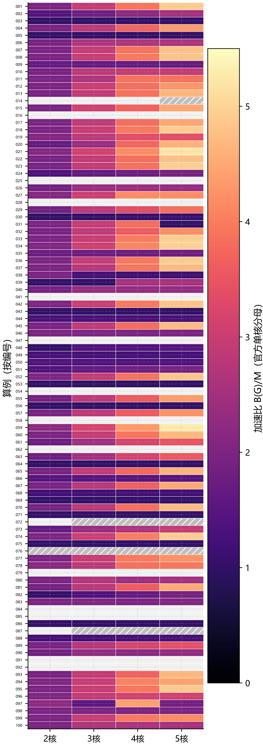
P1 加速比热图 — Batch A farmer-q1-v3 (官方单核分母; 斜纹=超时/失败)
