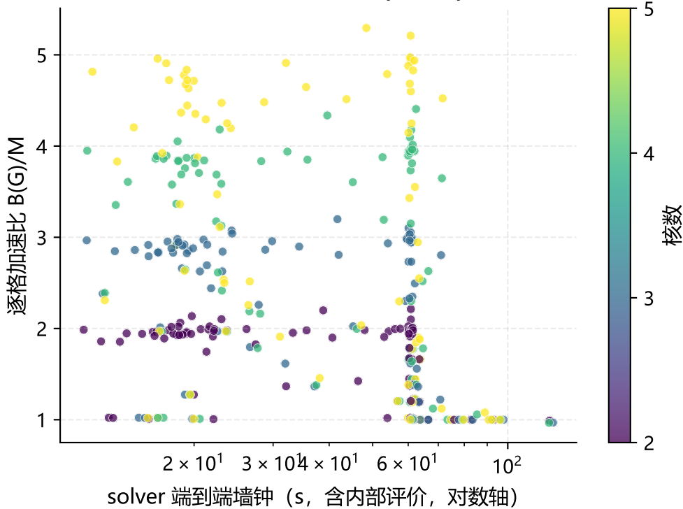
P1 求解耗时 vs 加速比 (334 格)
