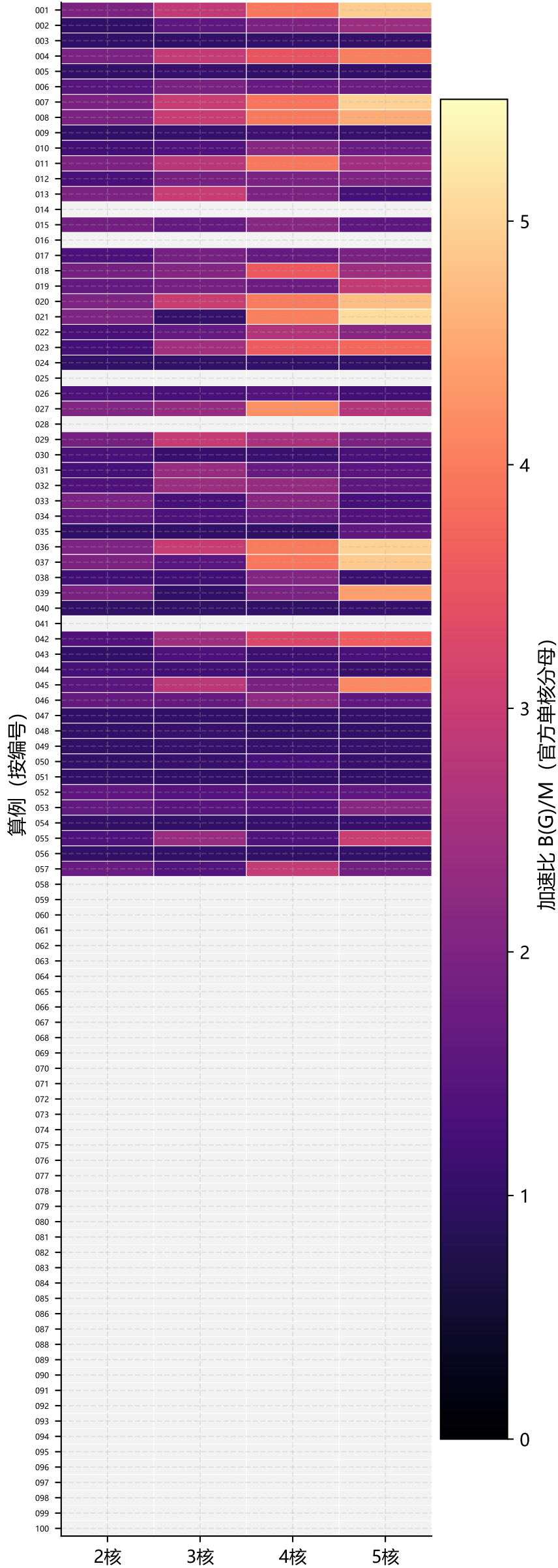
P2 加速比热图 — Batch B lyx-p123-multicore (12:17Z 快照, 灰斜纹=超时/失败, 浅格=未覆盖)
