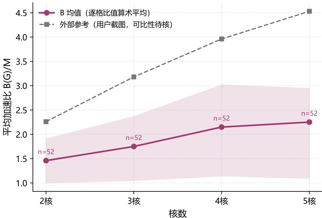
P2 平均加速比 vs 核数 (Batch B)
