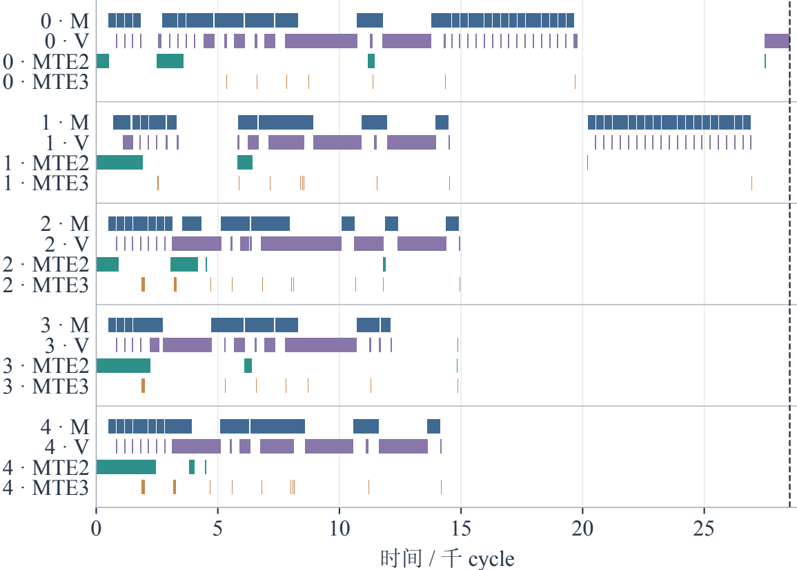
(b) 每核四条 Pipe 的实际占用区间
