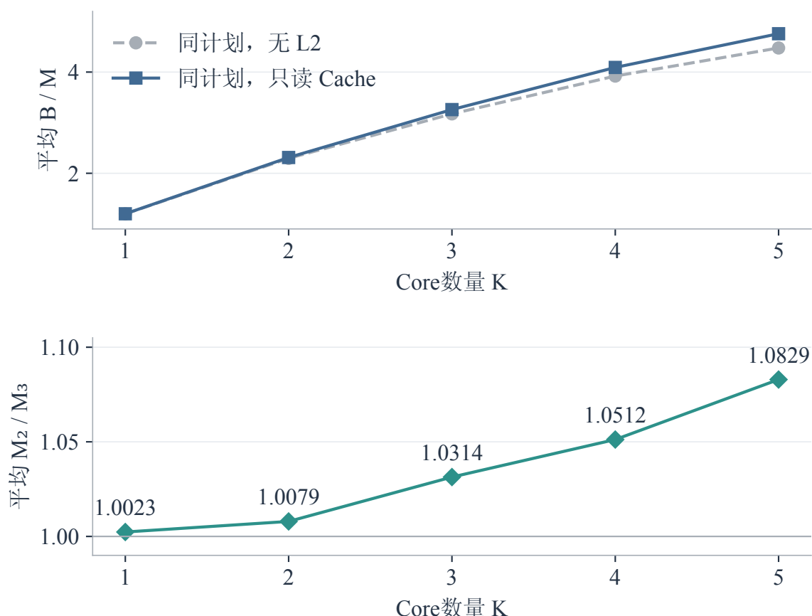
图 6.8-1 问题三的保持方案不变的配对评价。上：无 L2 与只读 Cache 的平均基线加速比；下：逐图 M_2/M_3 的均值，每种核心数量包含 100 对结果。
