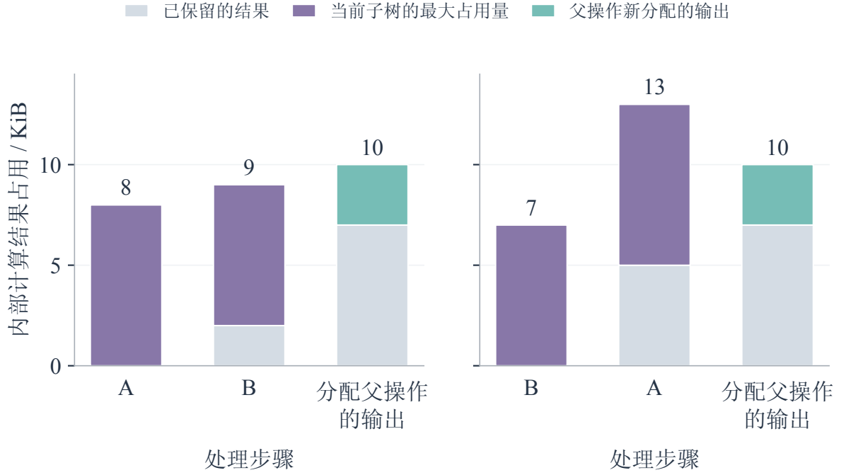
图 6.2-1 两种子树处理顺序的内部结果占用。左：先 A 后 B，峰值 10 KiB；右：先 B 后 A，峰值 13 KiB。横轴为处理步骤，不是模拟时钟；数字为第 6 章的公式示例。
