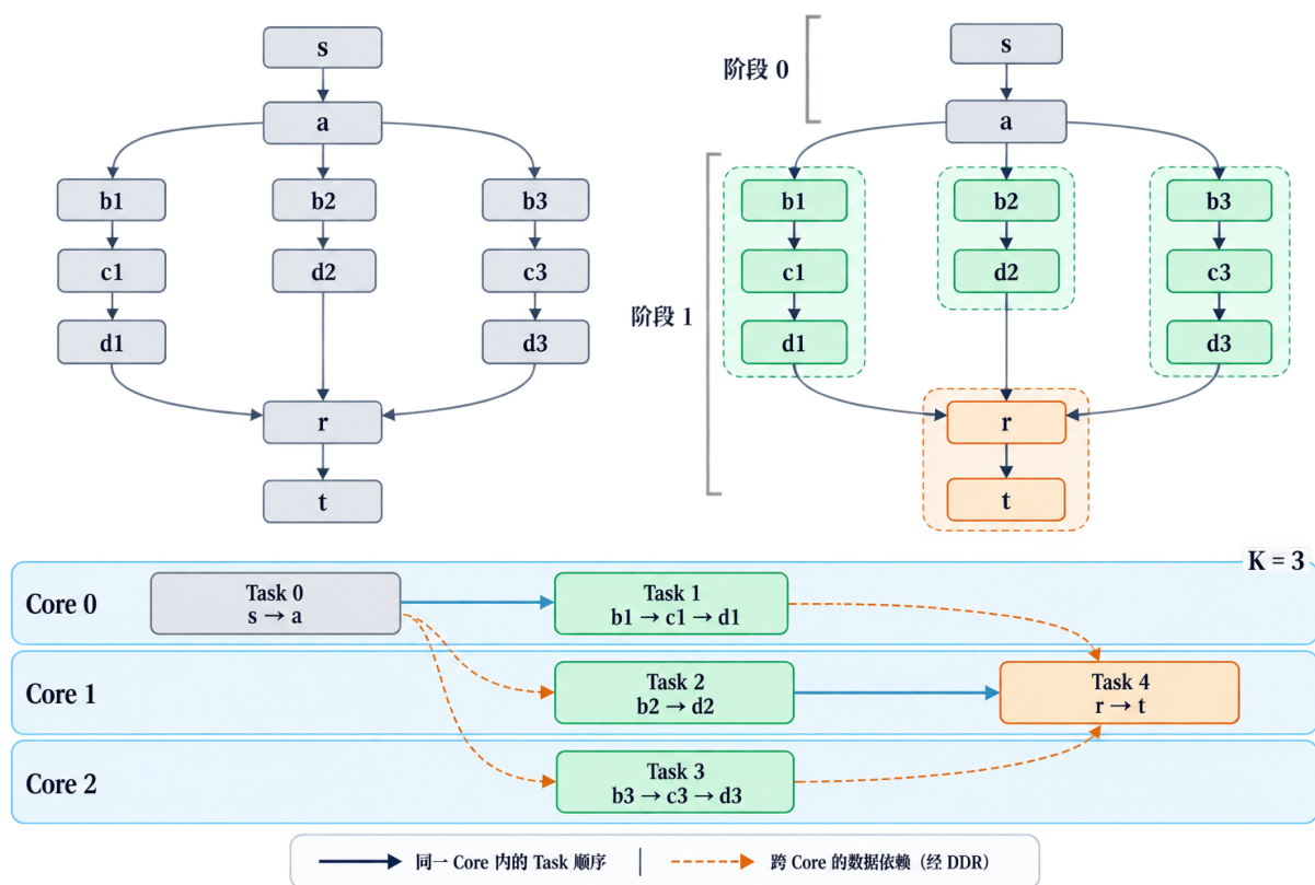
图 4.2 分叉—汇合结构的阶段划分与计算任务分配。左上为原始有向无环图，右上为阶段及节点分组，下方为三个核心上的任务分配与顺序。本图为结构示例，条块宽度与水平间距不表示执行时间。
