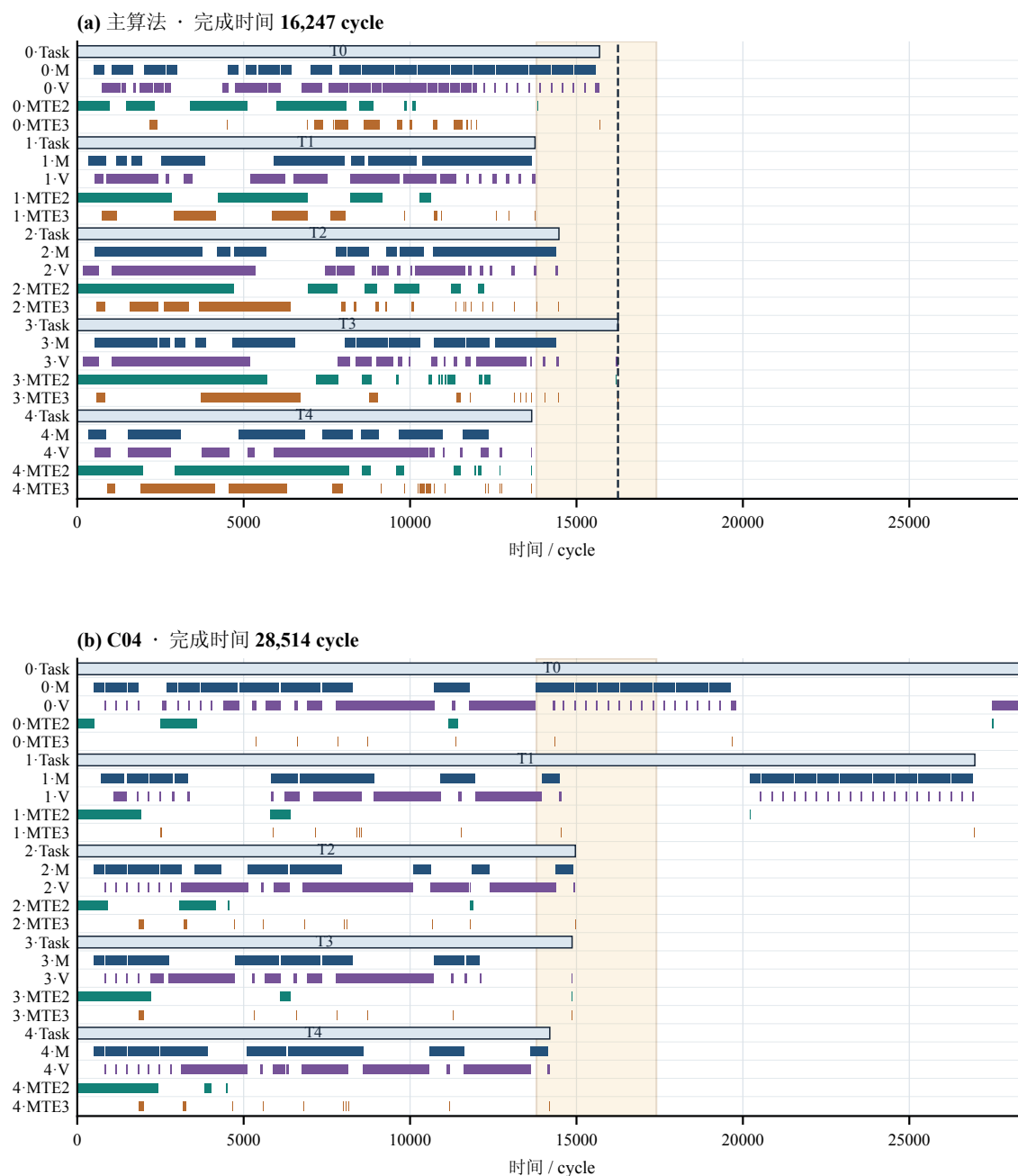
图 5-8 主算法与对照方案的完整执行时序
