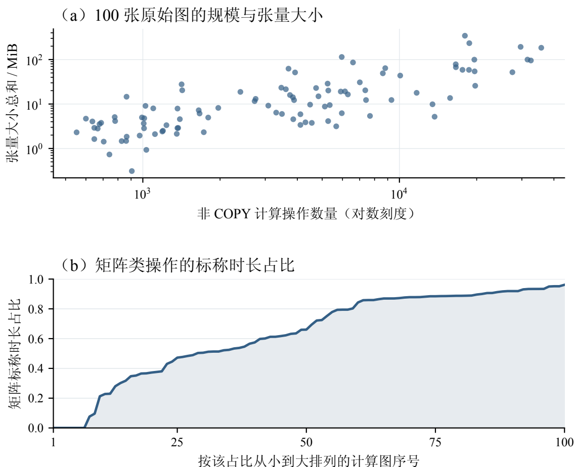
图 7-1 基准计算图规模与操作时长构成
