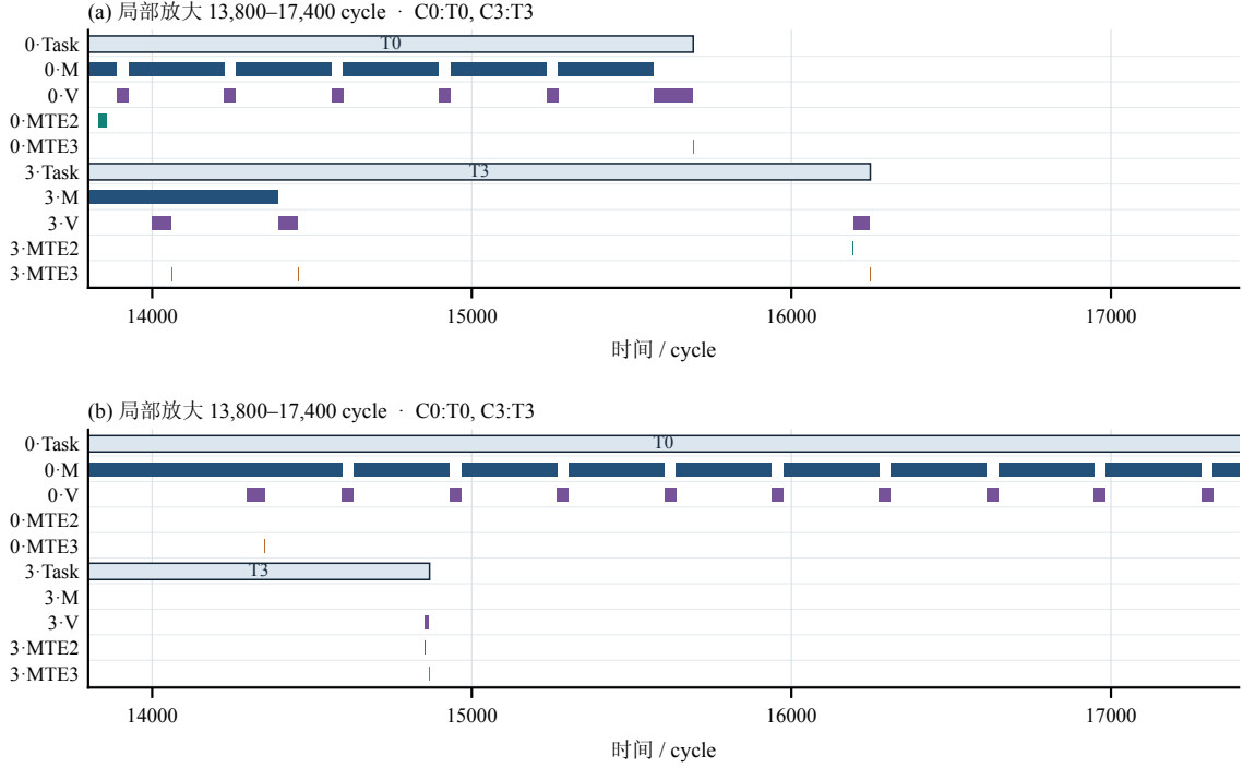
图 5-9 主算法与对照方案的局部执行时序
