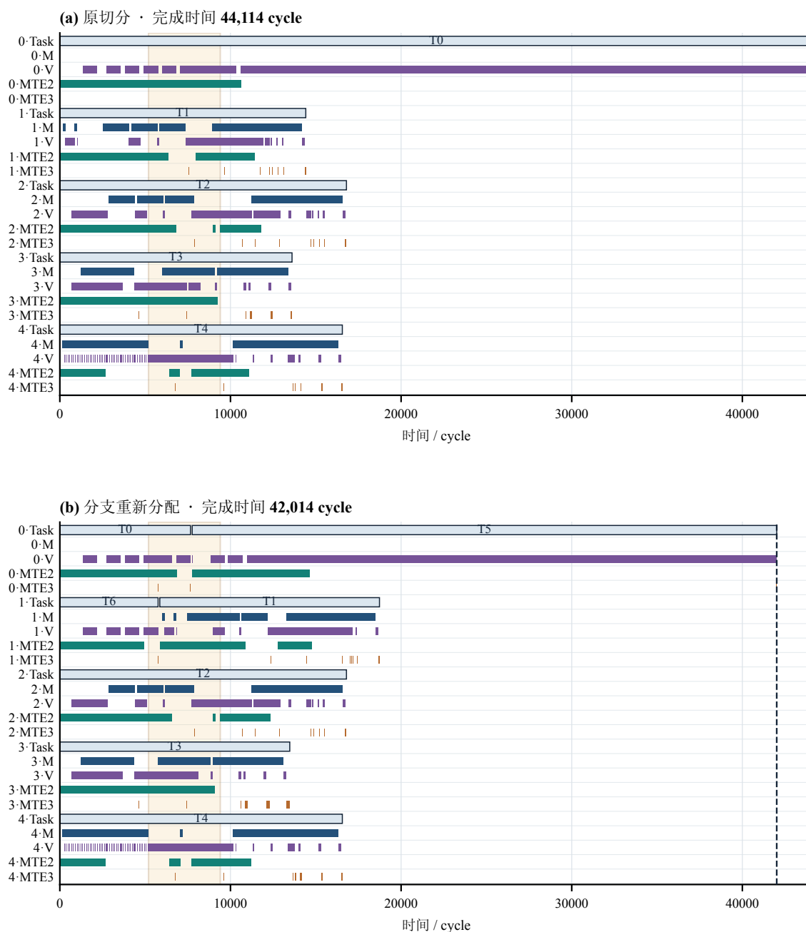
图 4-5 分支重分配前后的完整执行时序
