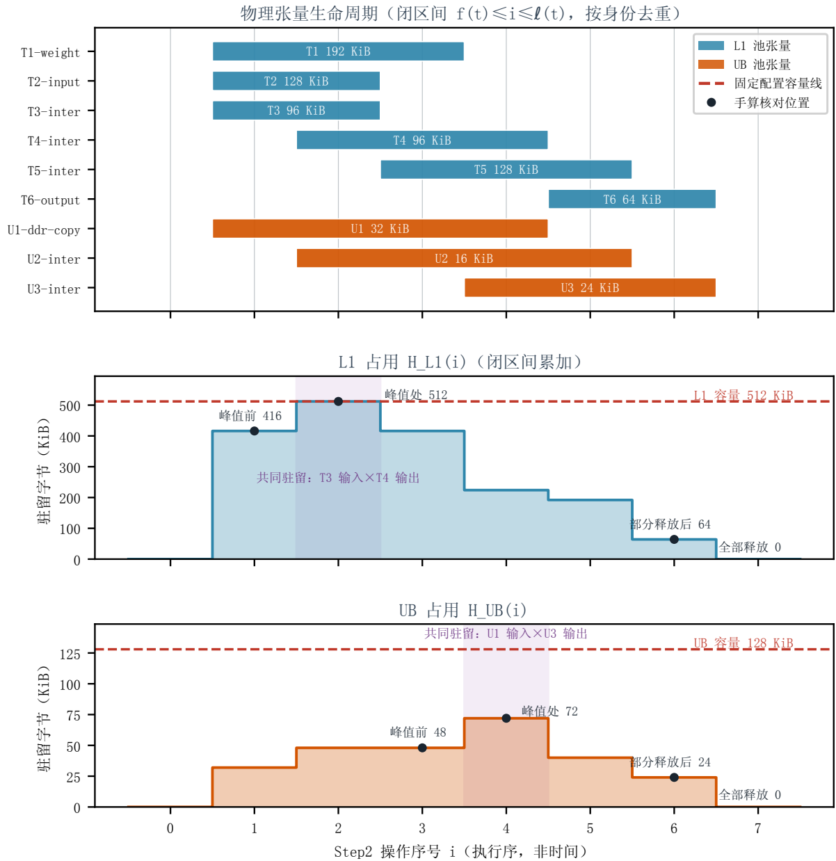
图 5-1 张量生命周期与片上存储占用
