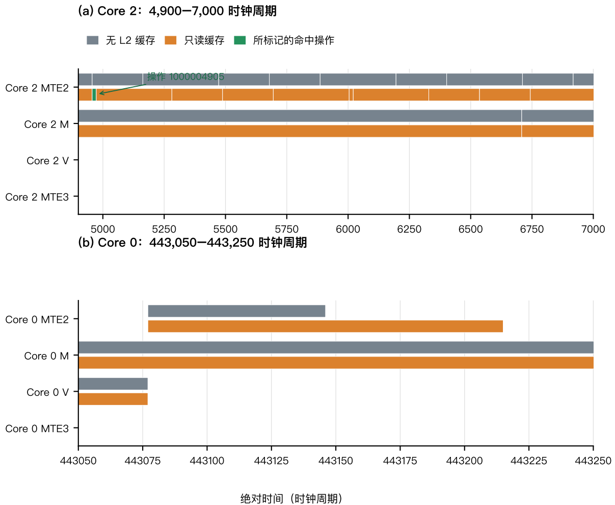
图 6-2 共享缓存开关对局部执行时序的影响
