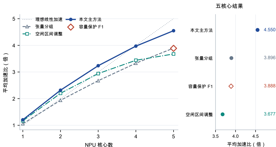
图 5-6 问题二各方法平均加速比对比
