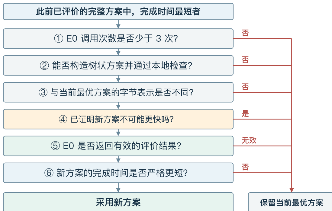
图 6-4 问题三子树排序与候选选优流程
