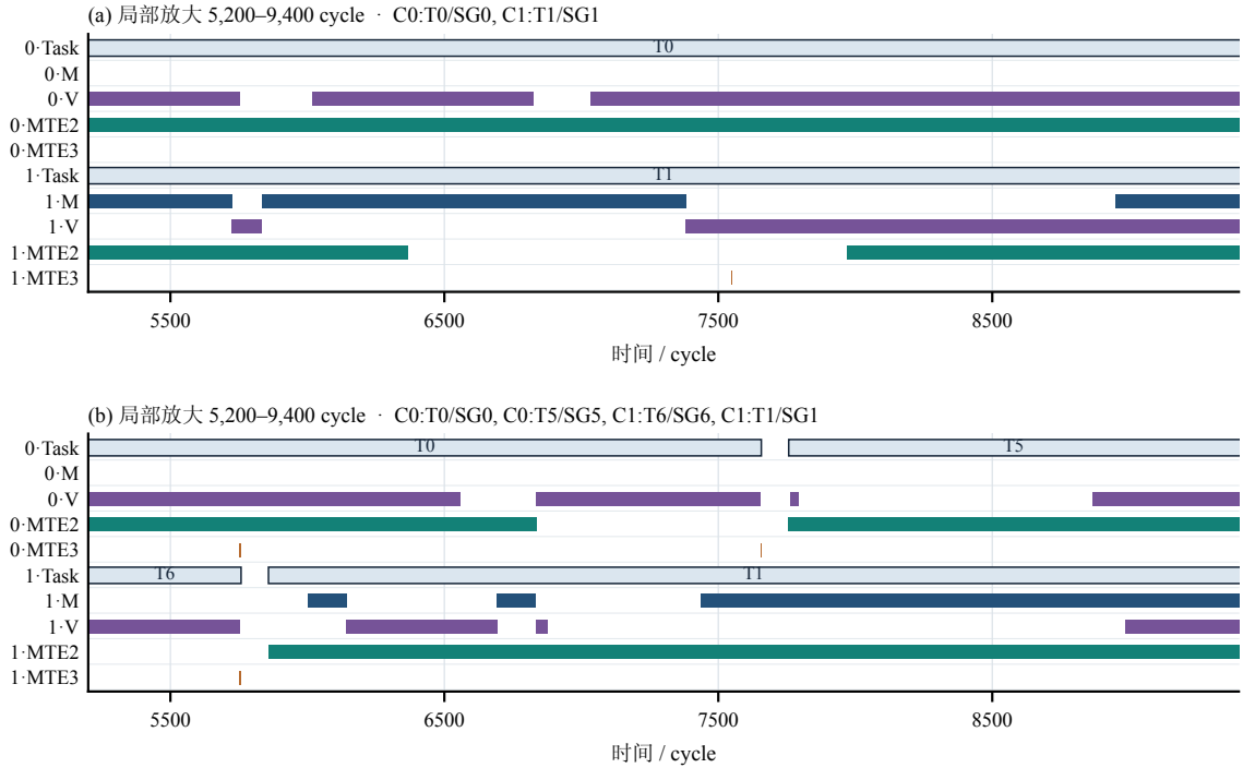
图 4-6 分支重分配前后的局部执行时序
