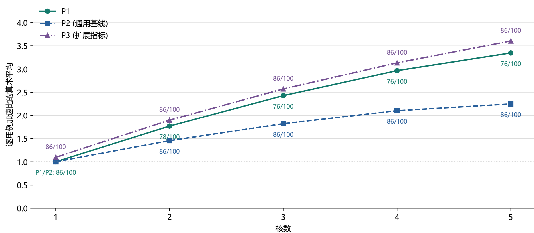
逐用例加速比的算术平均
