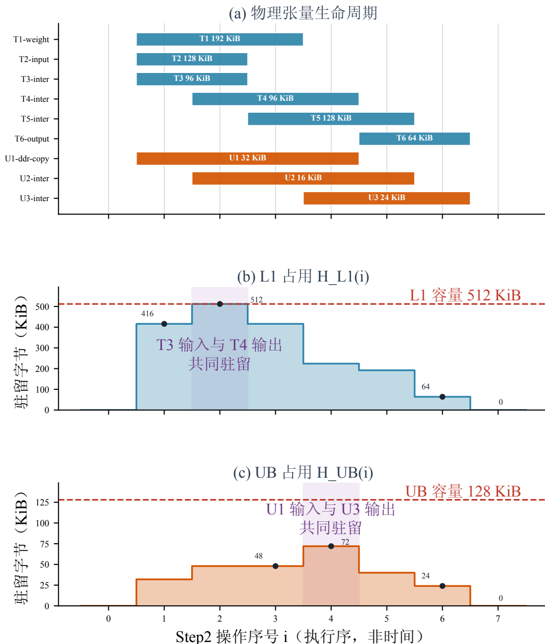
图 5.1-1 单核心张量生命周期与片上私有缓存容量占用手算示例。上部展示 9 个物理张量在闭区间 [f(t), \ell(t)] 内的驻留条带（如 T_6 = [5, 6] 与 U_3 = [4, 6] ）；中部与下部展示基于模仿 Step 2 静态编译操作序号下的 L1 Buffer（容量 512 KiB，步骤 2 达峰值 512 KiB）与 Unified Buffer（容量 128 KiB，步骤 4 达峰值 72 KiB）存储占用阶梯曲线，说明输入与输出张量在操作边界共同驻留对局部容量峰值的影响。图中无官方 spill 事件记录且未绘制溢出事件，横轴为静态操作序号而非微架构物理执行周期。
