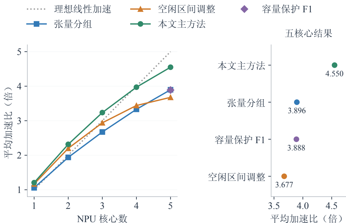
图 5.4-2 问题二四种固定方法的多核平均加速比对比。左侧展示三种全覆盖方法在 1~5 核心下的逐图平均加速比曲线与容量保护 F1 方法在 5 核心下的独立测试点，灰色点线为理想线性加速参照；右侧为 5 核心场景下各方法的横向对比展开。
