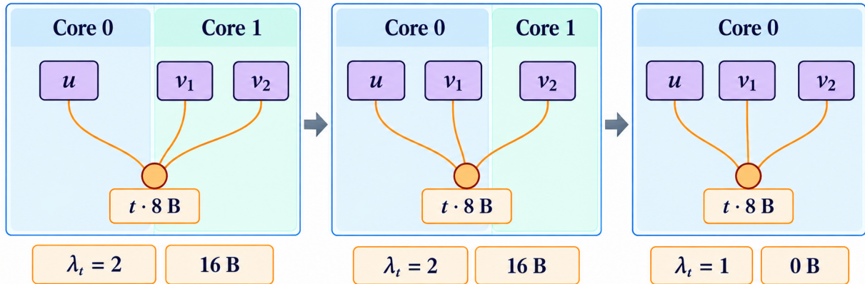
图 5.2-1 同一张量的计算操作分配。图中 u 生成 t ， v_1, v_2 读取 t ； \lambda_t 表示这三个操作所在的不同核心数量。16 B、16 B、0 B 仅统计该张量的边界复制，线条只表示集合关联。
