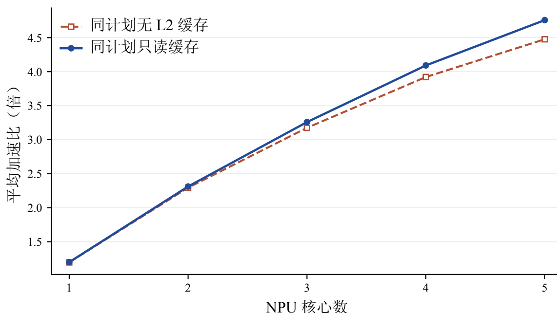
图 6-5 问题三共享缓存开关下的平均加速比
