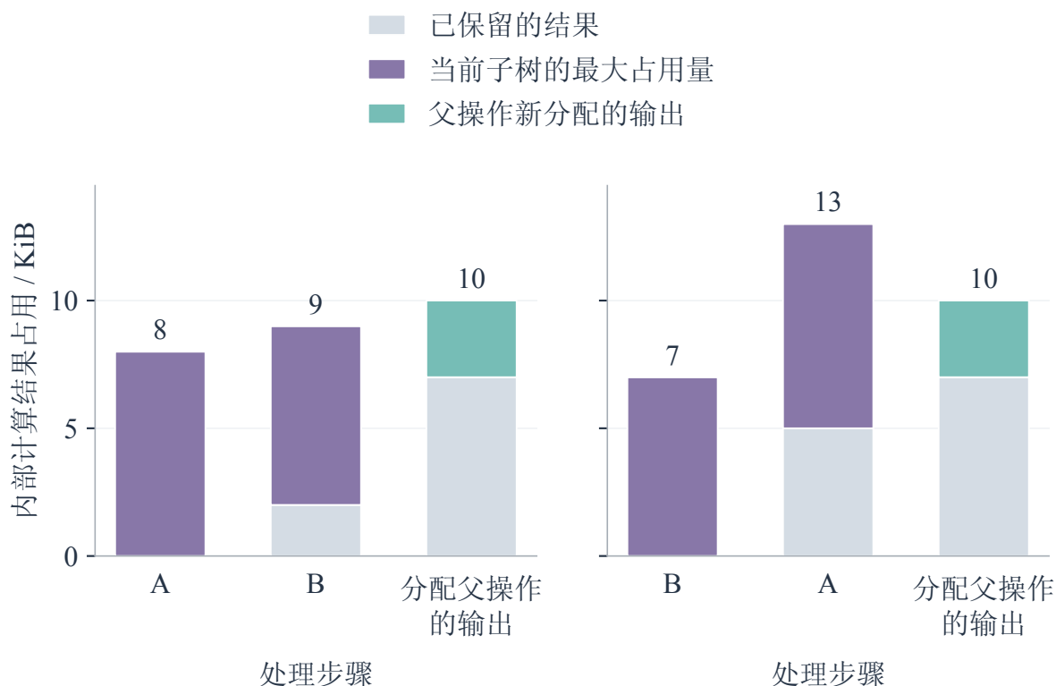
图 6-3 子树处理顺序与中间结果存储占用
