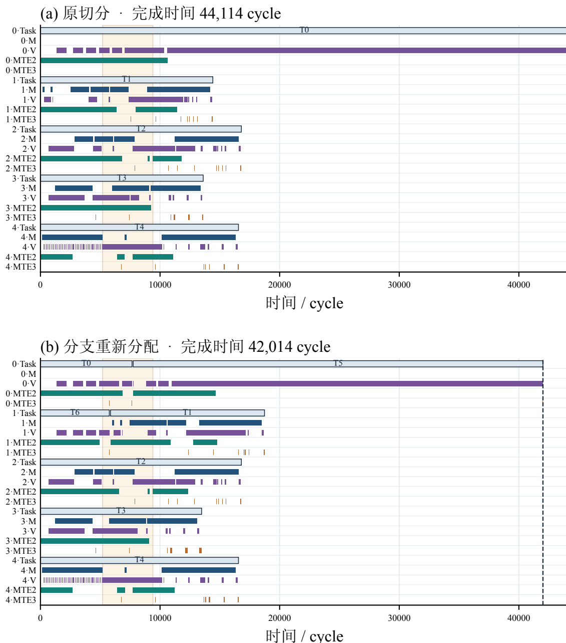
图 4-5 分支重分配前后的完整执行时序
