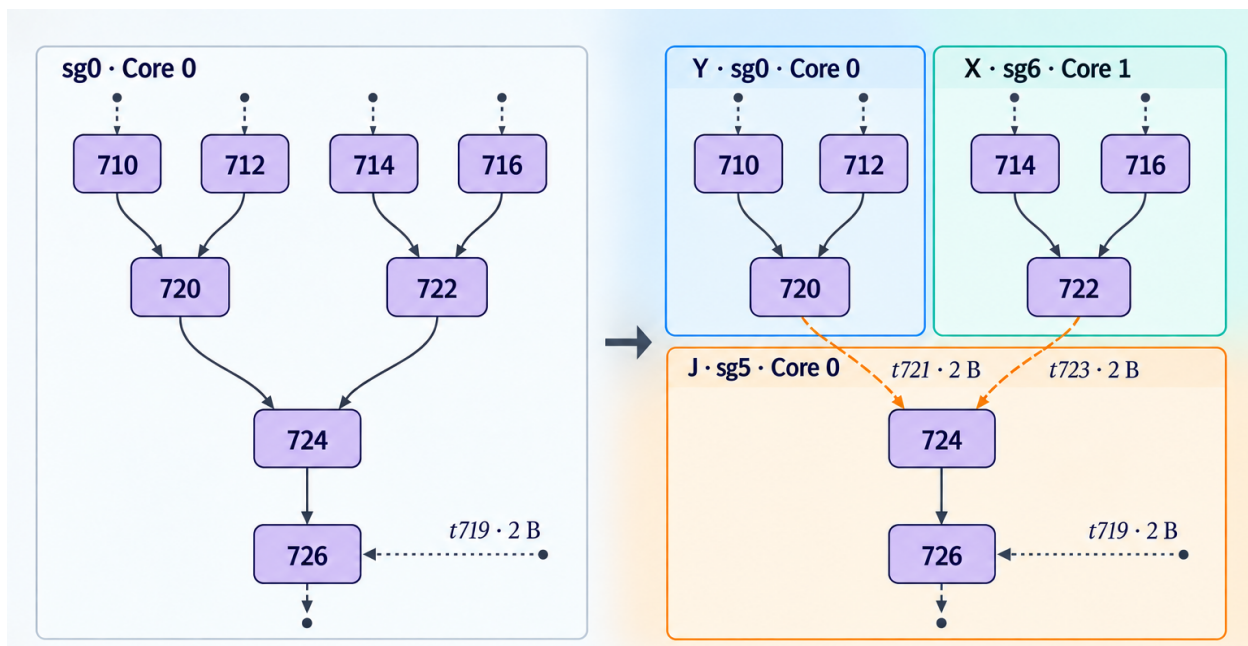
图 4-3 独立分支重分配前后的切分结构
