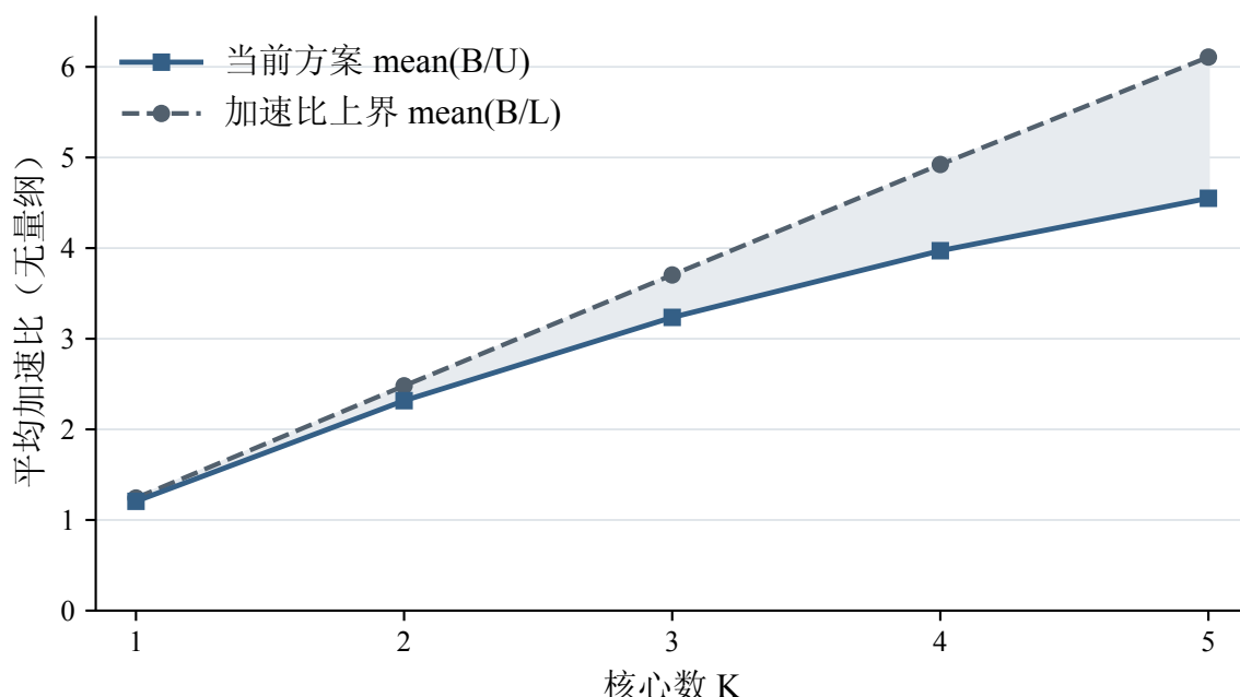
图 7-3 平均加速比与理论上界对比
