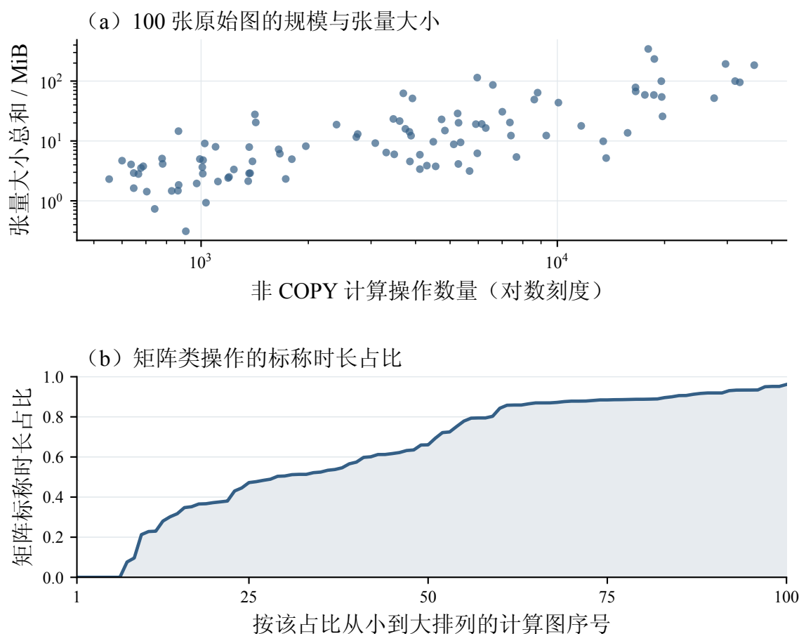
图 7-1 基准计算图规模与操作时长构成
