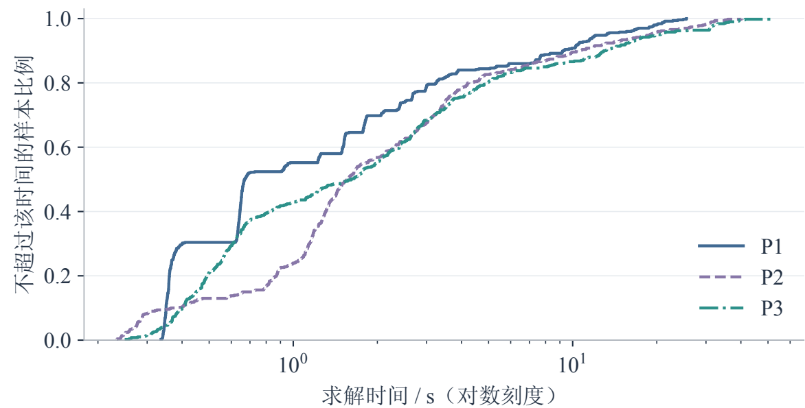
图 7-2 三问端到端求解耗时累积分布
