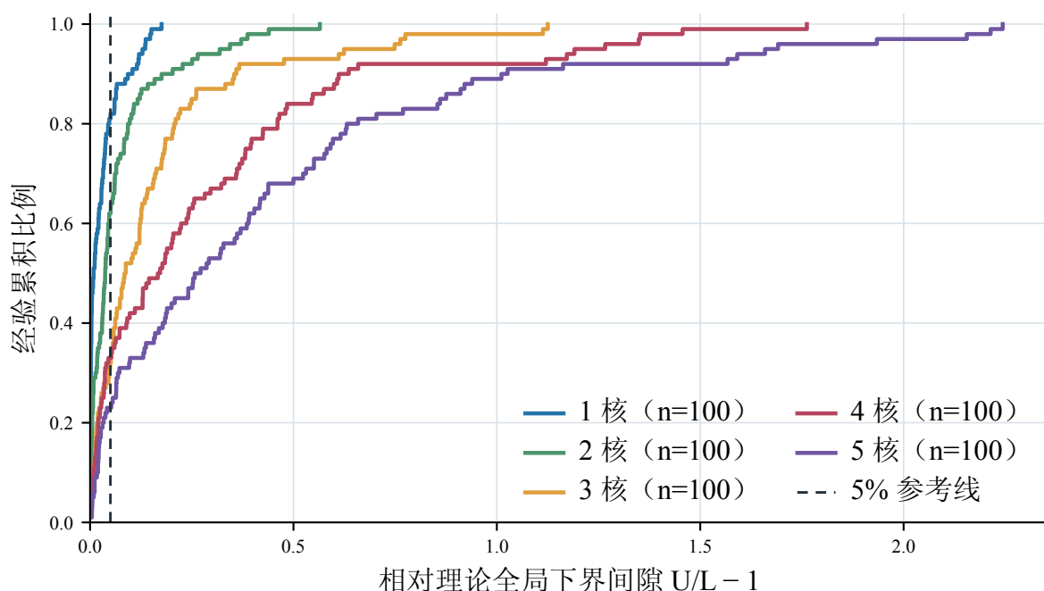
图 7-4 问题二相对下界间隙累积分布
