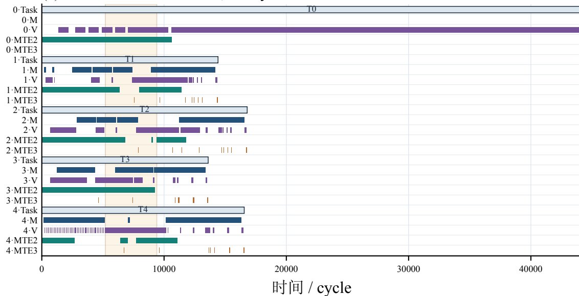
(a) 原切分 · 完成时间 44,114 cycle
