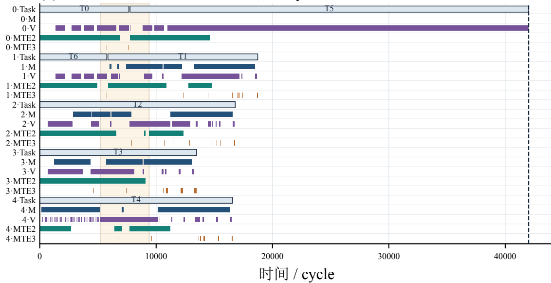
(b) 分支重新分配 · 完成时间 42,014 cycle
