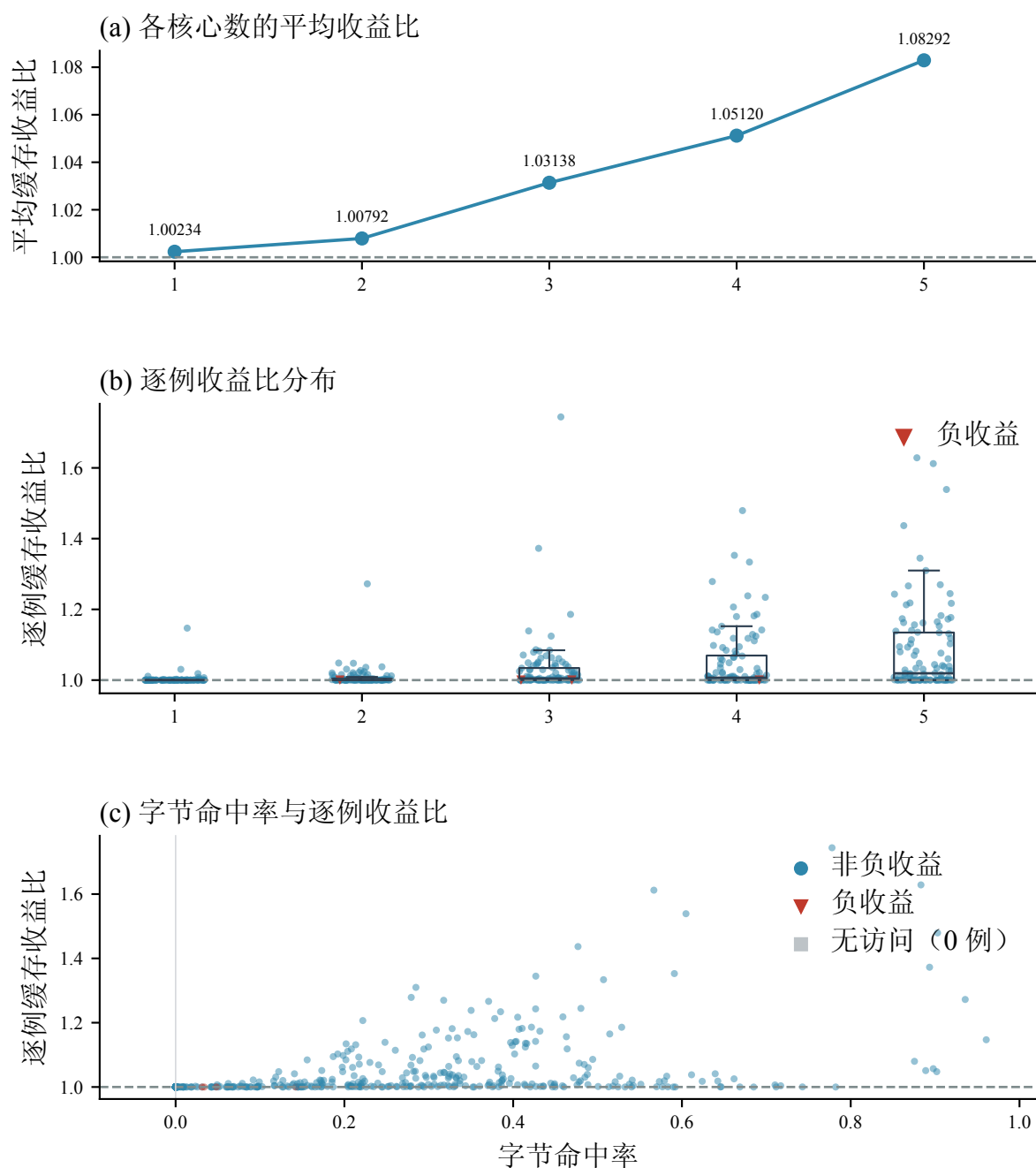
图 6-6 共享缓存加速比与字节命中率分布
