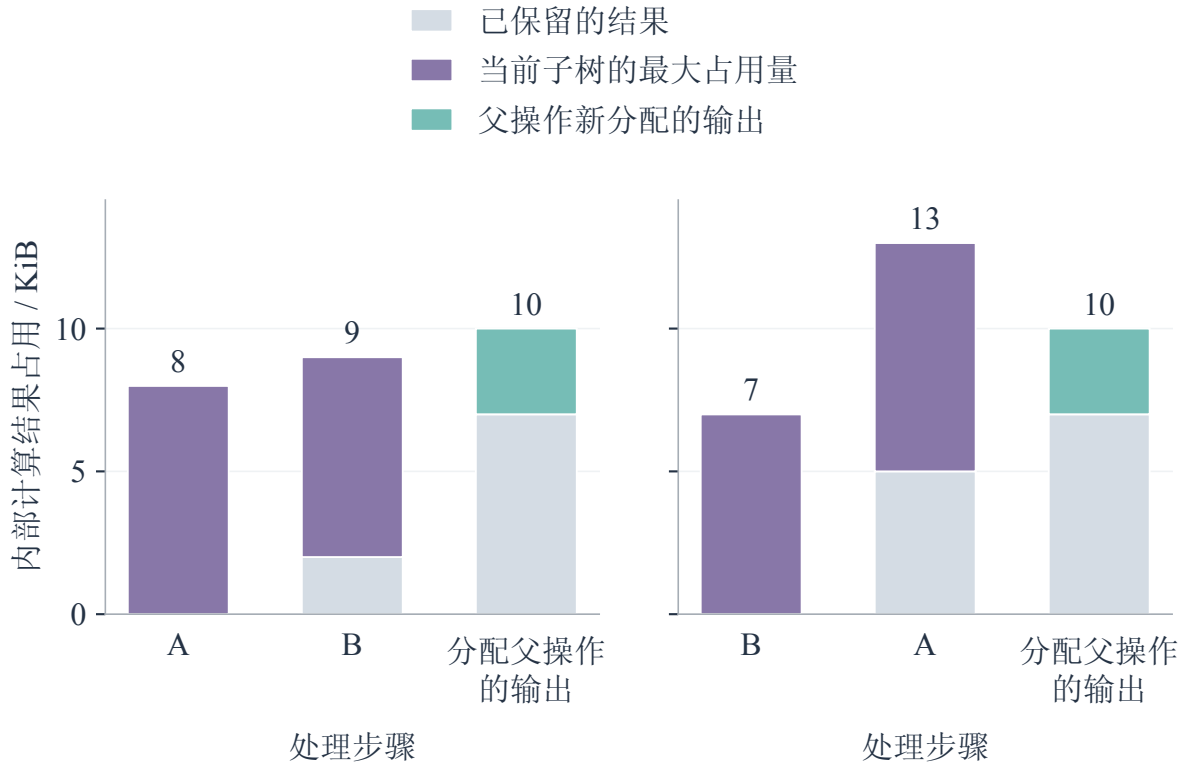
图 6-3 子树处理顺序与中间结果存储占用
