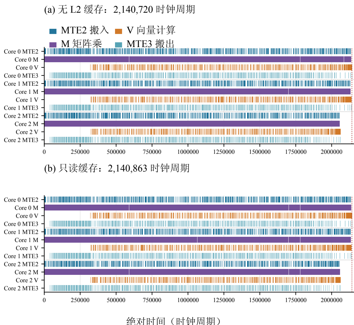
图 6-1 共享缓存开关对完整执行时序的影响
