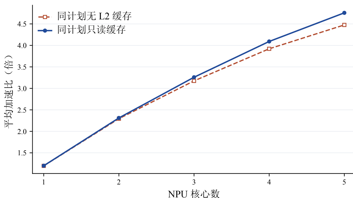
图 6-5 问题三共享缓存开关下的平均加速比
