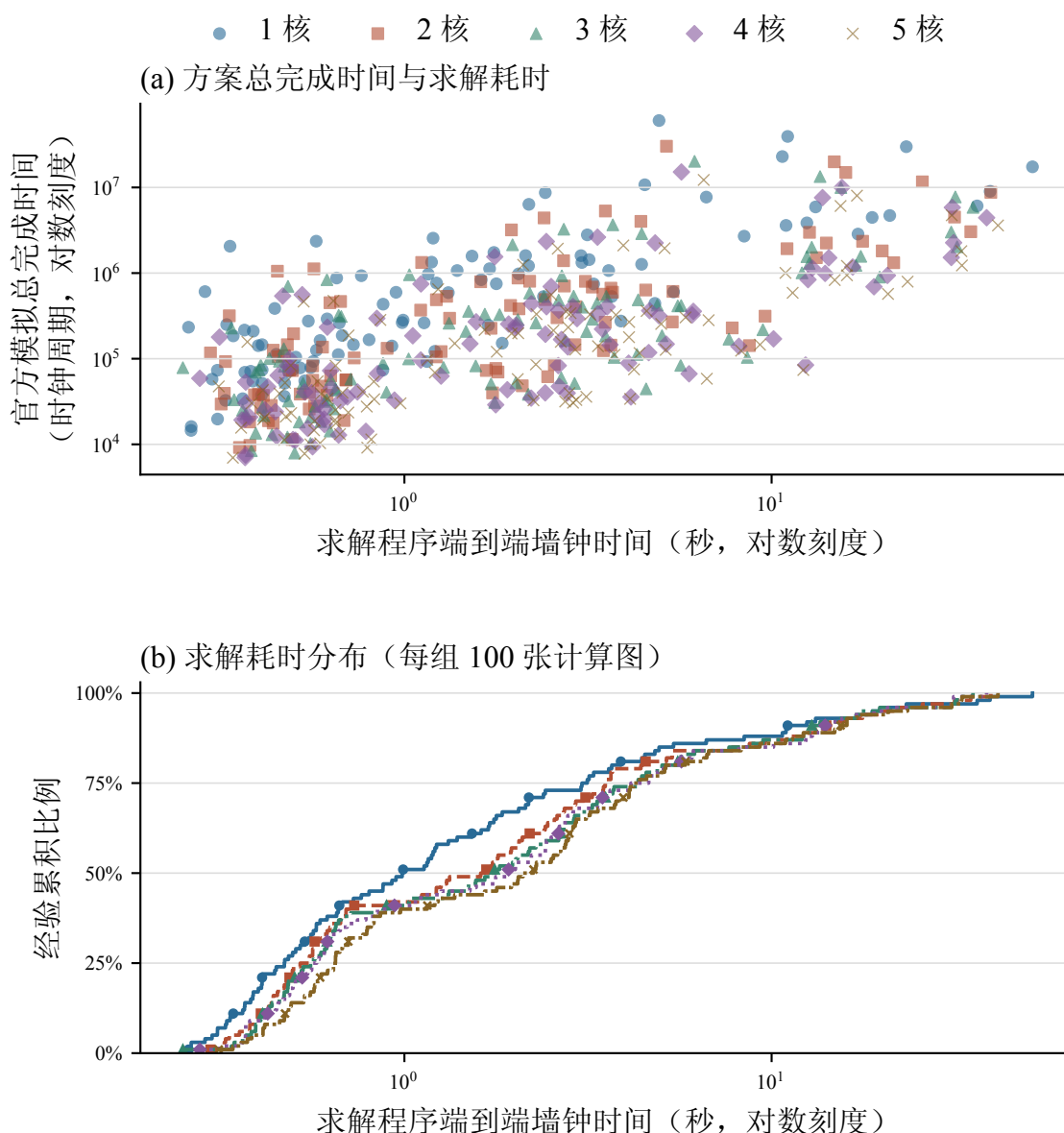
图 6-7 问题三方案完成时间与求解耗时分布
