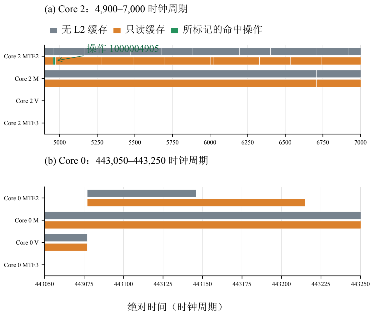
图 6-2 共享缓存开关对局部执行时序的影响
