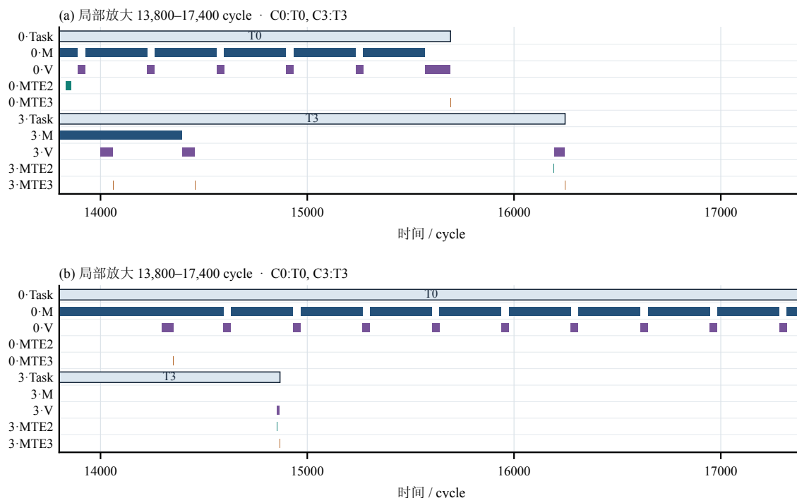
图 5.7-2 case_019 (5 核心) 两方案在关键局部时间窗 (13,800 至 17,400 cycles) 的时序放大对比。展示主算法与 C04 在 Core 0 (C0:T0) 及 Core 3 (C3:T3) 等任务上的流水线事件分布。图中未着色空白区域仅客观反映对应流水线未记录操作占用, 不作未经事件级归因分析的机理臆测。
