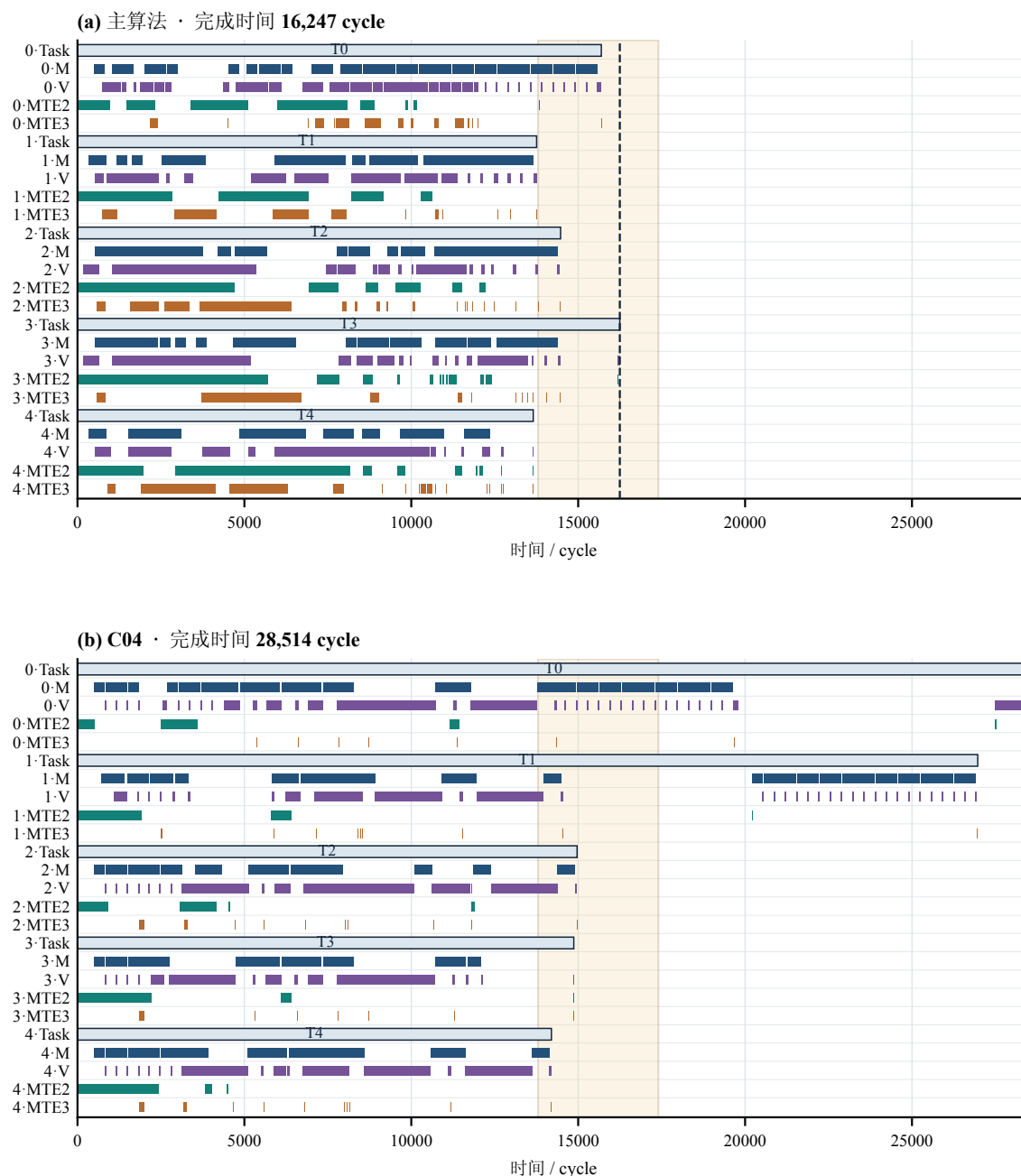
图 5.7-1 case_019（5 核心）主算法与 C04 对照方案全景执行时序对比。展示两方案在全流程时间尺度（0 至 28,514 cycles）下各核心 Task 与 Pipe 活跃区间；C04 方案无容量不足引起的缓存换入换出（spill 为 0），但完成时间（28,514 cycles）劣于主算法（16,247 cycles）。
