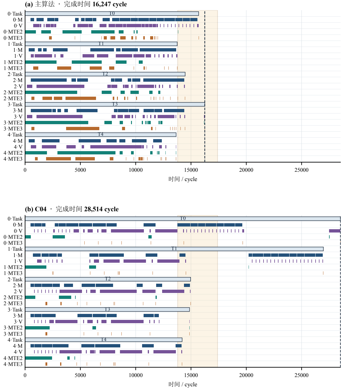
图 5.7-1 case_019 (5 核心) 主算法与 C04 对照方案全景执行时序对比。展示两方案在全流程时间尺度 (0 至 28,514 cycles) 下各核心 Task 与 Pipe 活跃区间；C04 方案无容量不足引起的缓存换入换出 (spill 为 0)，但完成时间 (28,514 cycles) 劣于主算法 (16,247 cycles)。
