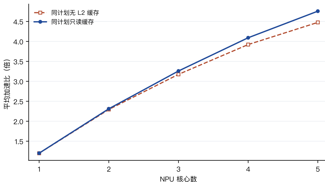
图 6.8-1 问题三开启只读 Cache 与同方案无 L2 运行的平均加速比对比。展示 1 至 5 核心下（每组 100 对同方案）逐用例计算 B/M 后的算术平均值；单核保留实际比值（无 L2 1.197143，只读 Cache 1.199760），不强制设定为 1。全量 500 对数据源于同计划机制对比，不替代独立优化的问题二主算法方案。
