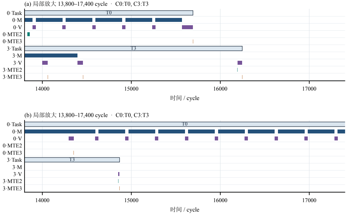
图 5.7-2 case_019 (5 核心) 两方案在关键局部时间窗 (13,800 至 17,400 cycles) 的时序放大对比。展示主算法与 C04 在 Core 0 (C0:T0) 及 Core 3 (C3:T3) 等任务上的流水线事件分布。图中未着色空白区域仅客观反映对应流水线未记录操作占用, 不作未经事件级归因分析的机理臆测。
