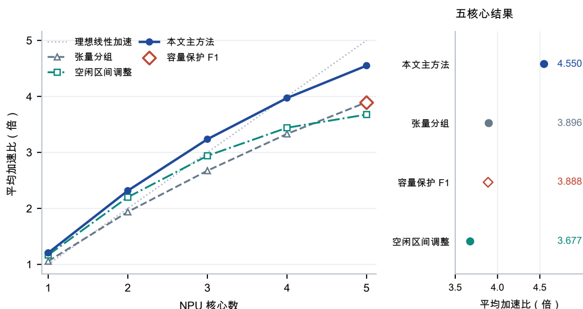
图 5.6-2 问题二四种固定方法的多核平均加速比对比。左侧展示三种全覆盖方法在 1~5 核心下的逐图平均加速比曲线与容量保护 F1 方法在 5 核心下的独立测试点，灰色点线为理想线性加速参照；右侧为 5 核心场景下各方法的横向对比展开。
