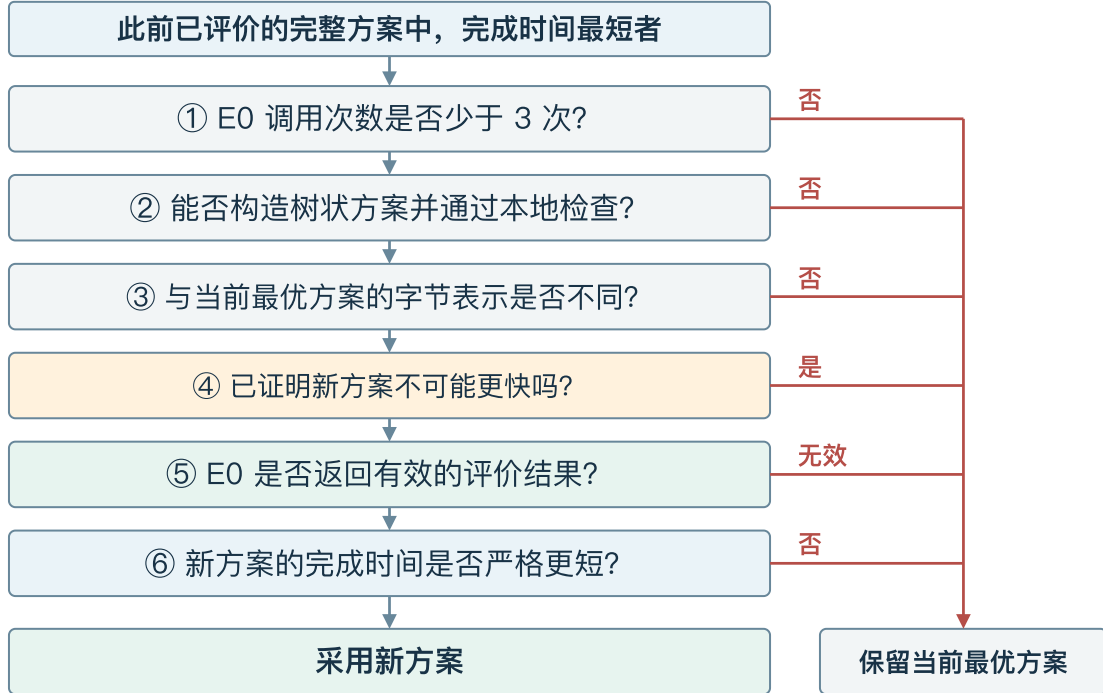
图 6.7-1 树状分支排序准则与完整候选方案的评测决策流程。展示基于指标差值 h_i - r_i 降序排定非交错子树次序以最小化树模型局部峰值存储，以及共享至多 3 次在线 E0 评测预算下的前置检查、与当前最优方案直接比对编码去重、下界剪枝与完成时间改善选优决策链。存储优化属于非交错树模型推导，不改变分核归属，非物理片上缓存实测峰值。
