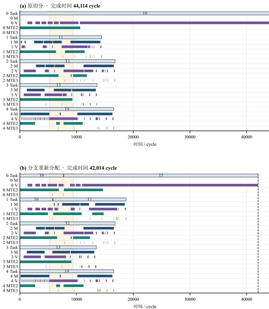
图 4.6-1 用例 case_026 在 5 核配置下重分配前后的完整执行时间线对比。基于官方模拟事件绘制，(a) 原始方案 Makespan 为 44,114 cycles，额外数据搬运量为 211,680 B；(b) 分支援助重分配后 Makespan 为 42,014 cycles，额外数据搬运量为 375,532 B。各核心 Task 行表示任务执行区间，M、V、MTE2、MTE3 分别表示四类硬件流水线的已记录操作区间，图中浅色区域标出 5,200–9,400 cycles 局部观察窗口。
