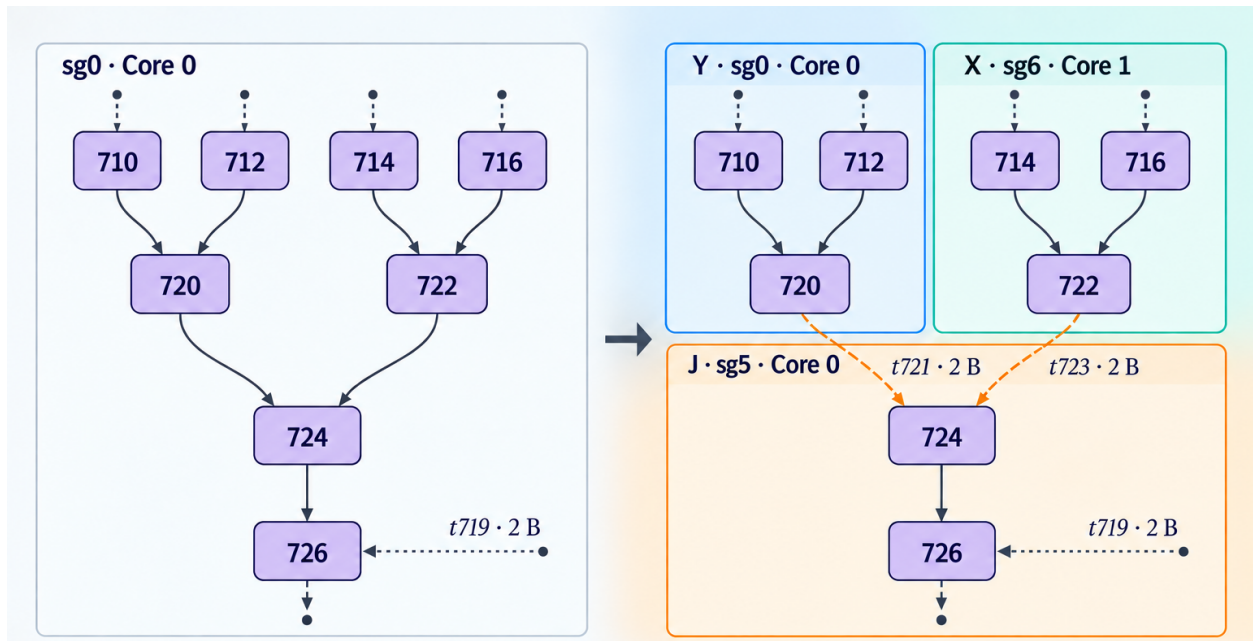
图 4.3-1 典型用例 case_026（5 Cores）独立分支重分配前后的切分结构映射。展示原始划分中 Core 0 上的超大任务解构为保留在 Core 0 上的独立支路 Y（算子 710、712、720）与汇合计算 J（算子 724、726），以及重分配至 Core 1 的导出独立支路 X（算子 714、716、722）。图中黑实线表示计算依赖，橙虚线表示跨子图数据依赖，点线端口表示连接至局部裁剪窗口外部的算子依赖（非孤立无依赖节点）。图示仅对应特定用例局部的 8 节点子图结构，不代表构造器处理的一般计算图全局结构。
