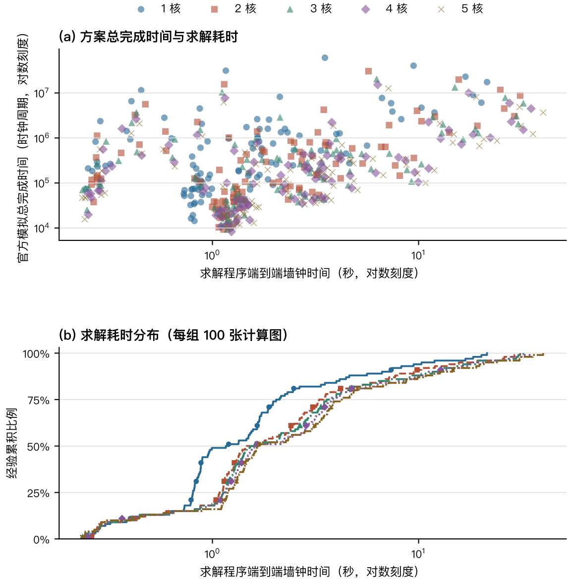
图 5.6-3 问题二主算法方案质量与求解耗时分布。上图展示 500 个测试组合在官方离散事件仿真下的 Makespan 与求解器端到端墙钟时间双对数散点分布；下图展示各核心数下（每组 100 用例）求解耗时的经验累积分布函数（ECDF）。评测在共享主机单 worker 进程环境下完成，计时涵盖子进程启动、图解析、在线 E2 评测与方案写出全流程。
