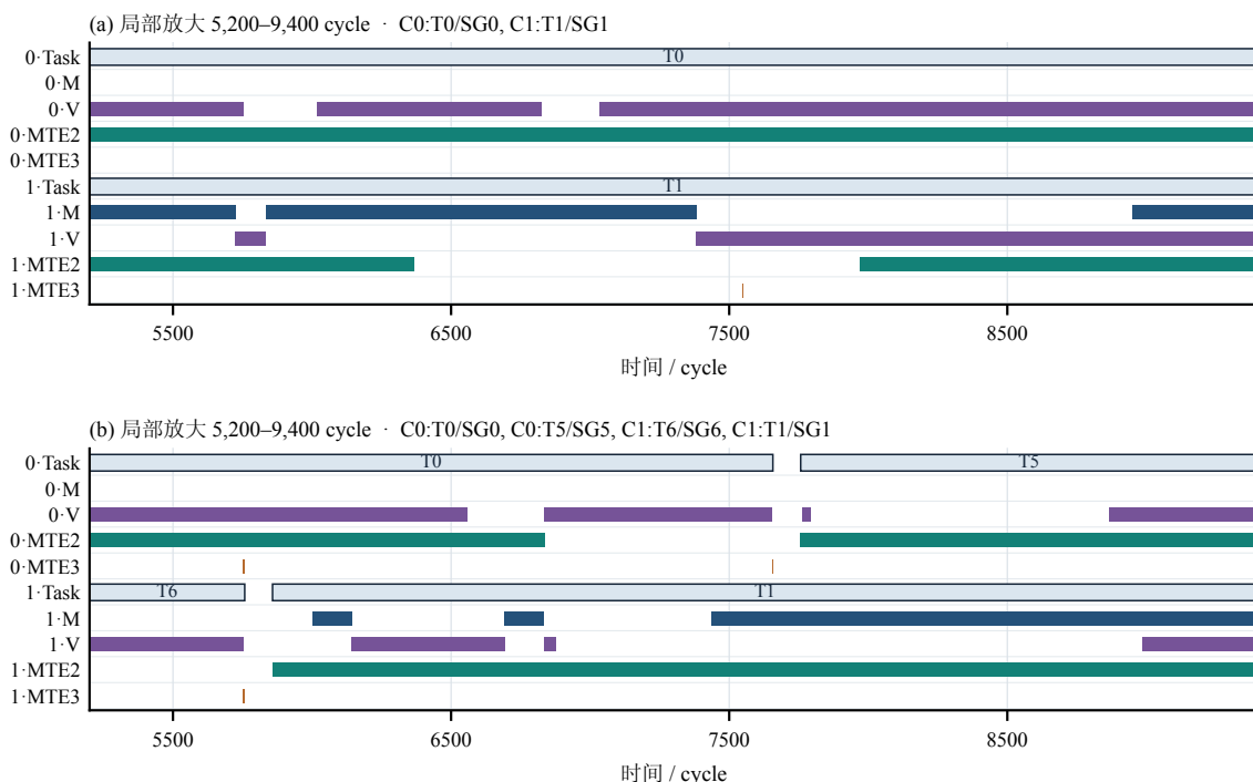
图 4.6-2 用例 case_026 在 5,200–9,400 cycles 窗口内的局部微架构流水线时序放大图（对应图 4.6-1 浅色区域）。展示核心 0 与核心 1 在该时段内的任务切换与各流水线操作事件分布。图中执行资源对应行的空白仅表示该时段未记录到流水线占用事件，不推定具体的外部等待原因。
