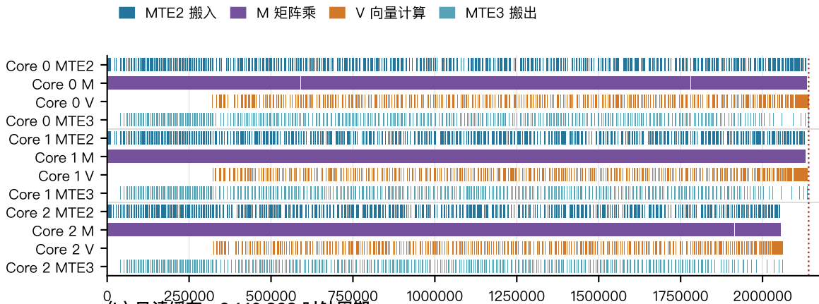
(b) 只读缓存: 2,140,863 时钟周期
