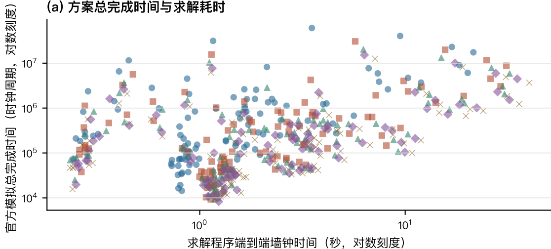
(a) 方案总完成时间与求解耗时
