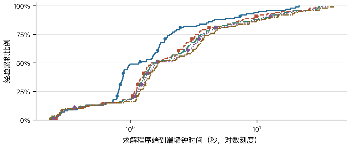
(b) 求解耗时分布 (每组 100 张计算图)
