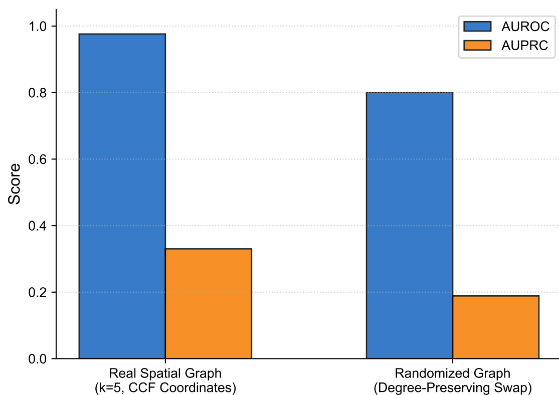
B. Discrimination (AUROC vs AUPRC)
