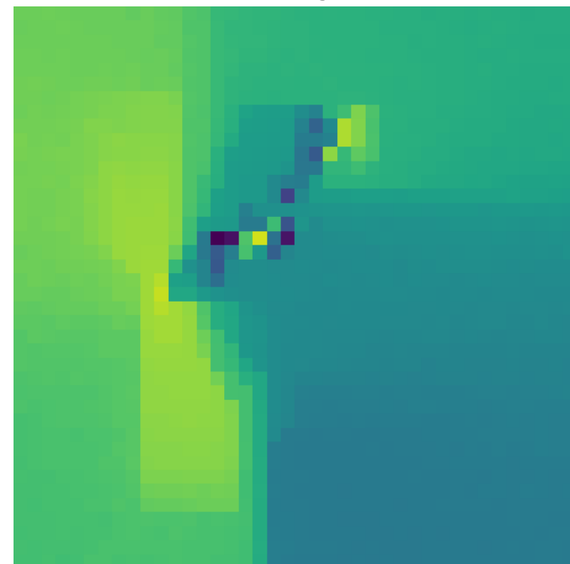
AVBD g_{12}
