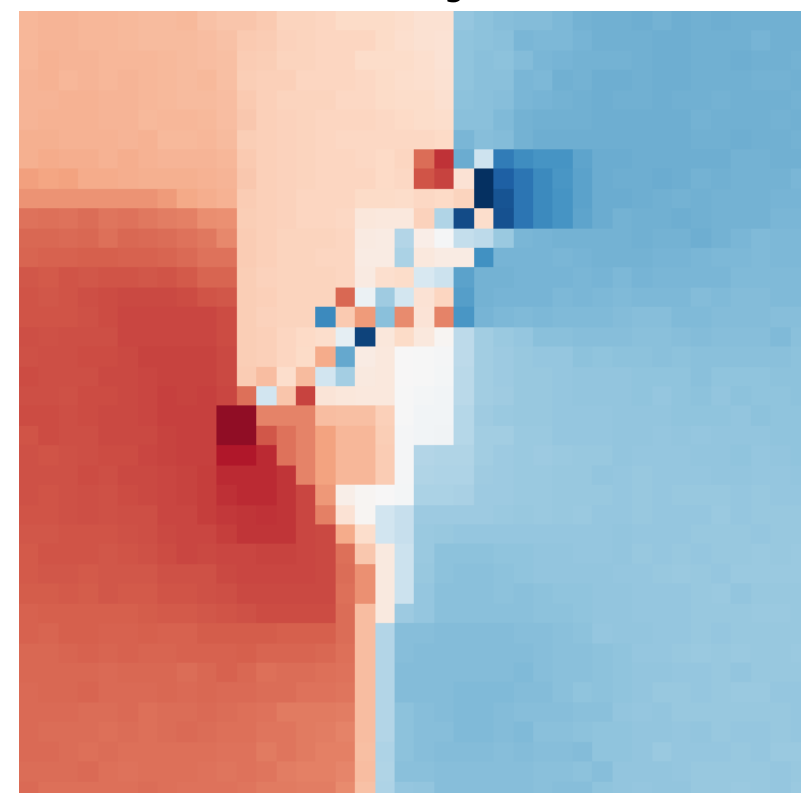
AVBD g_{22}
