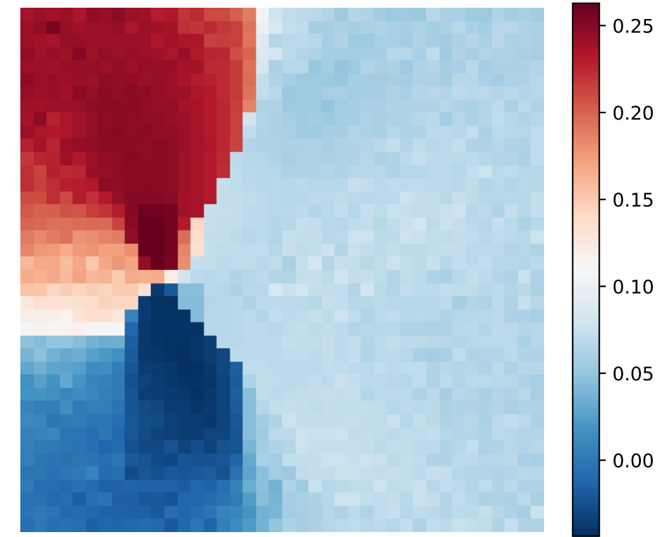
AVBD b_1
