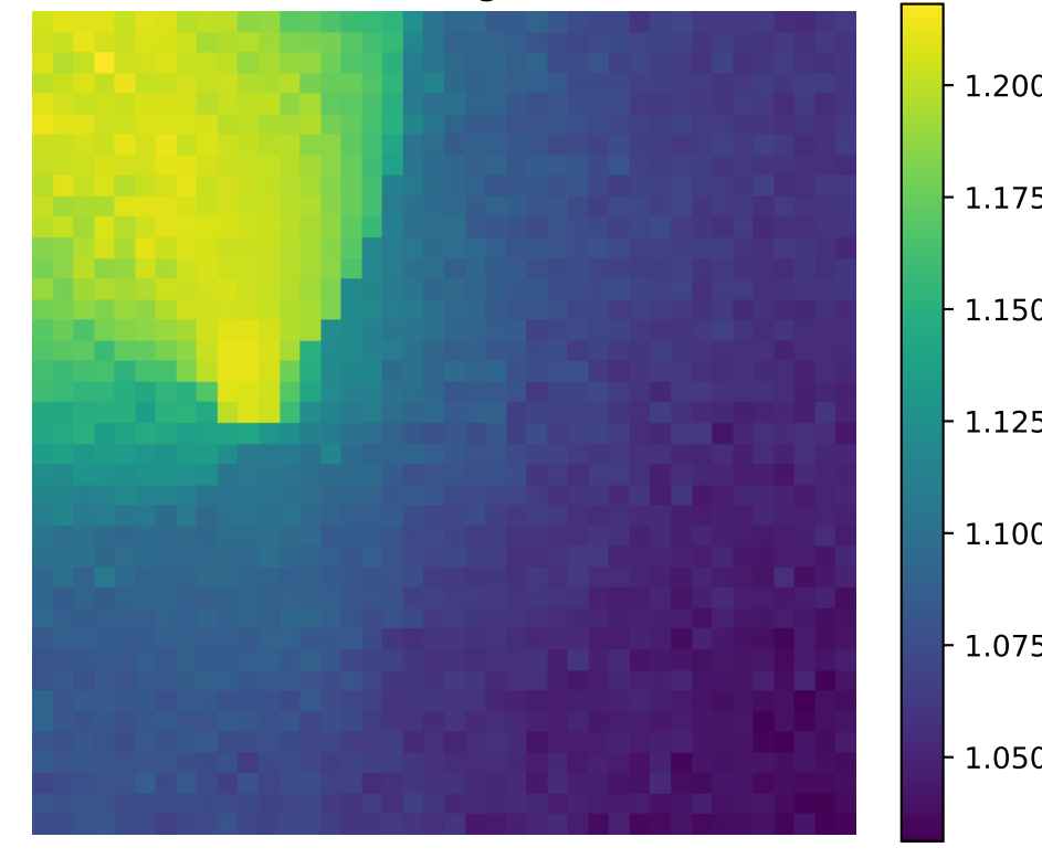
AVBD g_{11}
