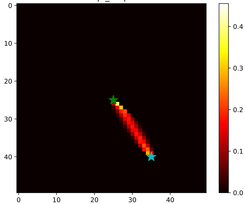
|\nabla_G L|
