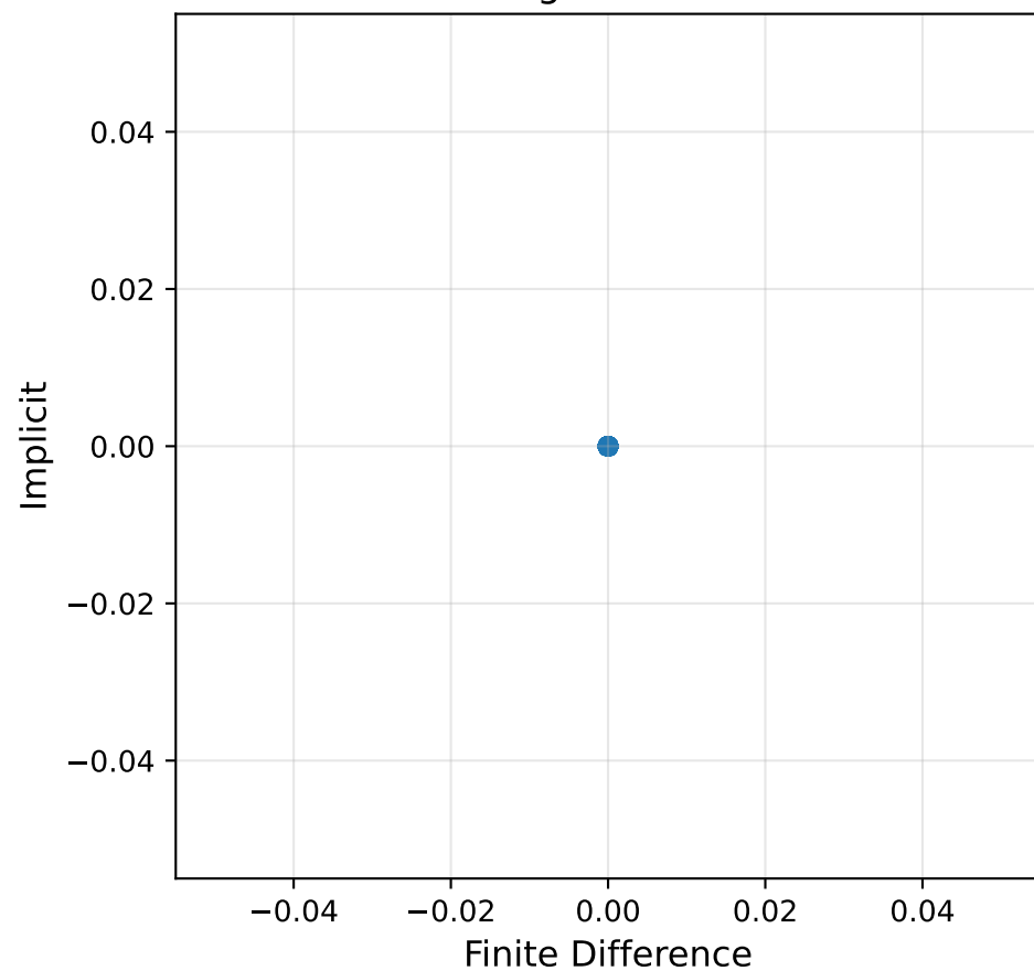
|\nabla_G L|
