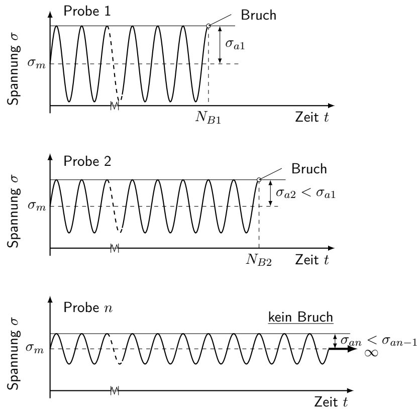
Abbildung 2.5.: Schwingungen der Einzelproben mit gleicher Mittelspannung und unterschiedlicher Spannungsamplitude (In Anlehnung an [8, Seite 273]).
