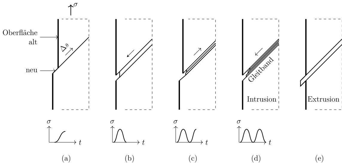
Abbildung 2.1.: Entstehung von Gleitbändern, sowie Intrusionen und Extrusionen infolge zyklischer Beanspruchung (In Anlehnung an [18, Seite 8]).
