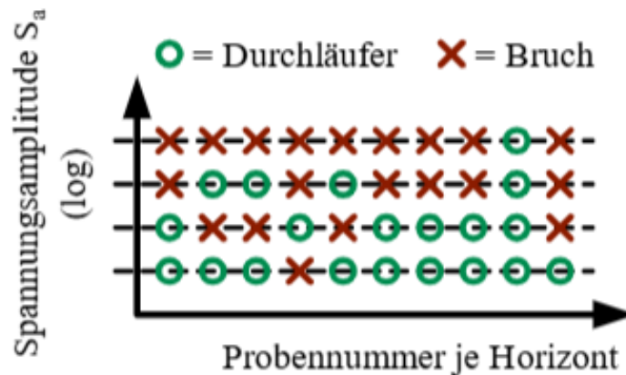
Abbildung 2.10.: Probit-Verfahren [17, Seite 36].
