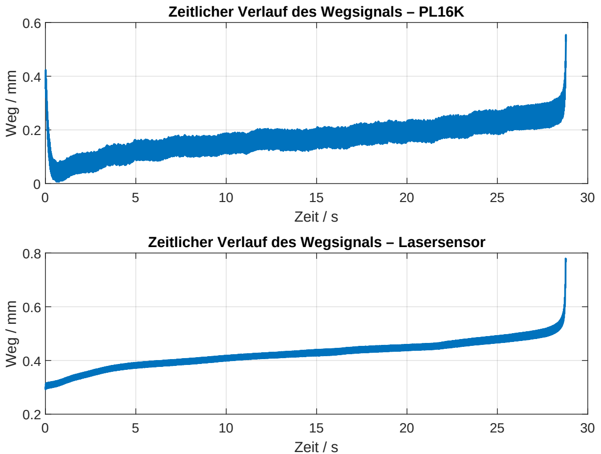
Abbildung 4.1.: Vergleich Wegsignal des Wegaufnehmers Lasersensor und des Wegaufnehmers PL16K.
