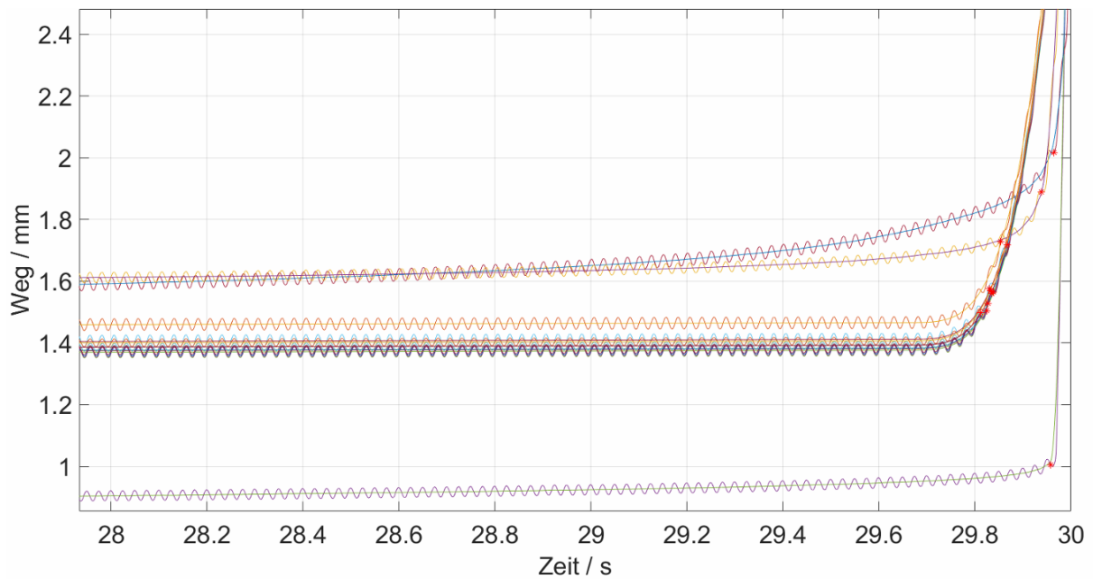
Abbildung 4.5.: Detailansicht zur Darstellung der Abbruchpunkte im Weg-Zeit-Diagramm der untersuchten Proben.
