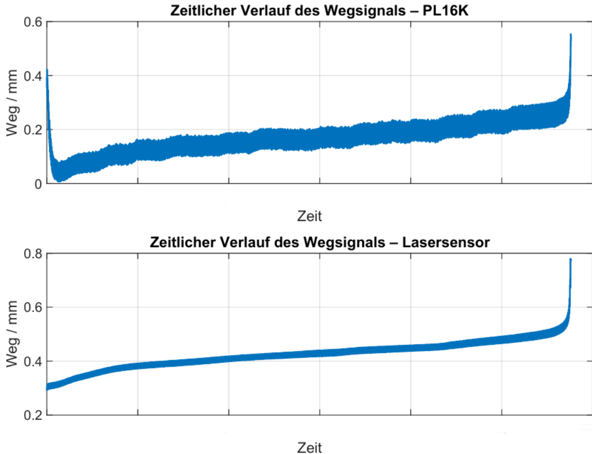
Abbildung 4.3.: Vergleich der Wegsignale des PL16K-Wegaufnehmers und des Lasersensors.
