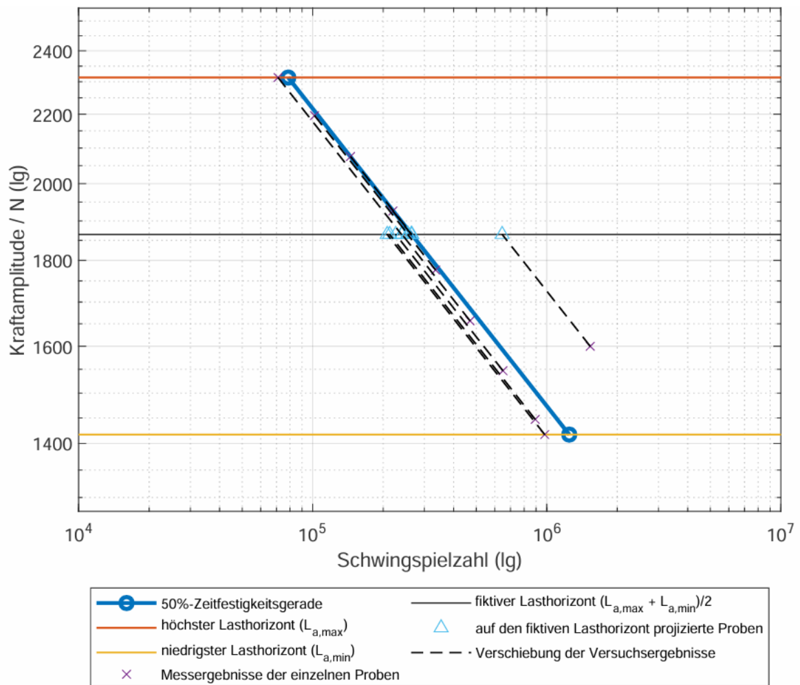
Abbildung 4.6.: Verschieben der Versuchsergebnisse auf einen gemeinsamen Lasthorizont (In Anlehnung an DIN 50100, Seite 56).
