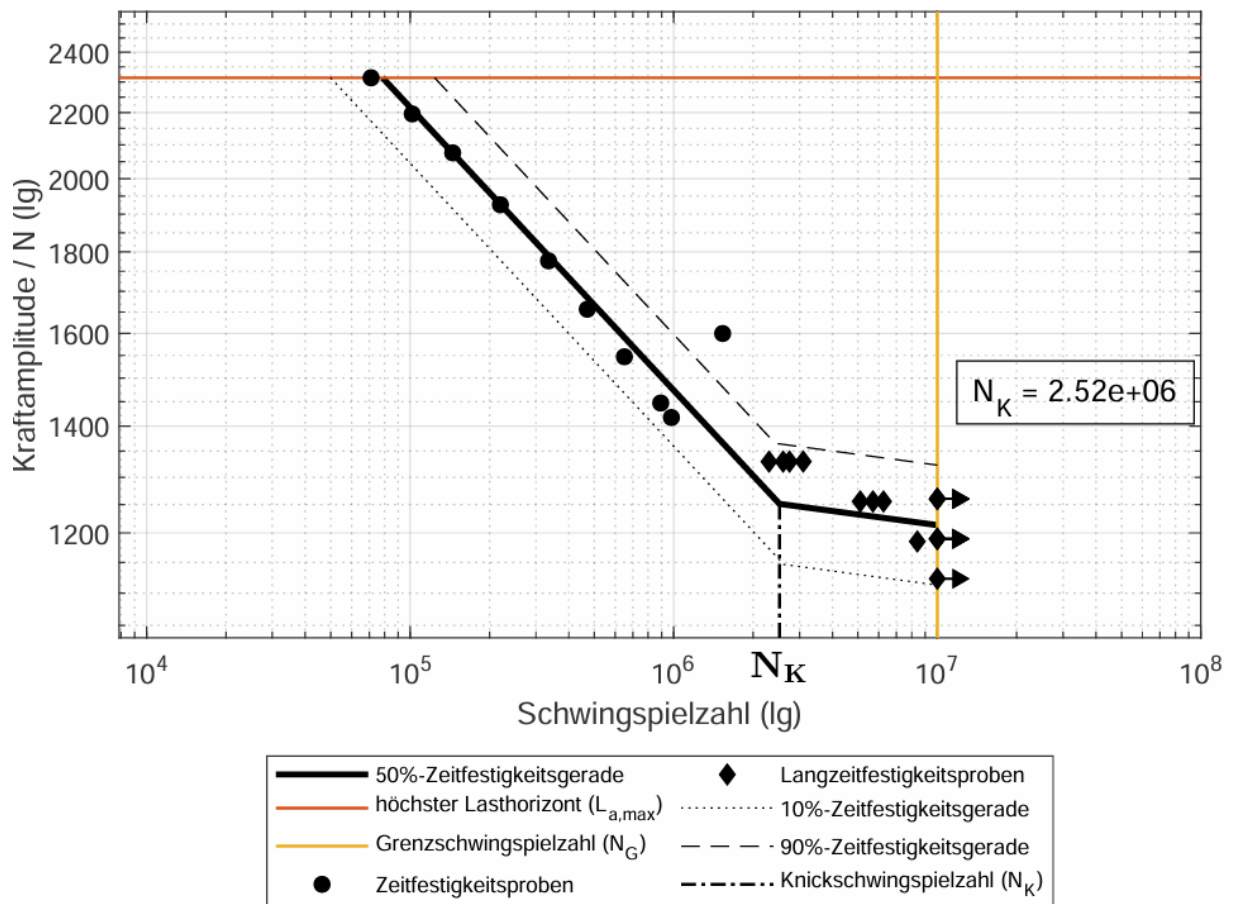
Abbildung 4.8.: Aus der MATLAB-Auswertung resultierende Wöhlerlinien des Auswertbeispiels
