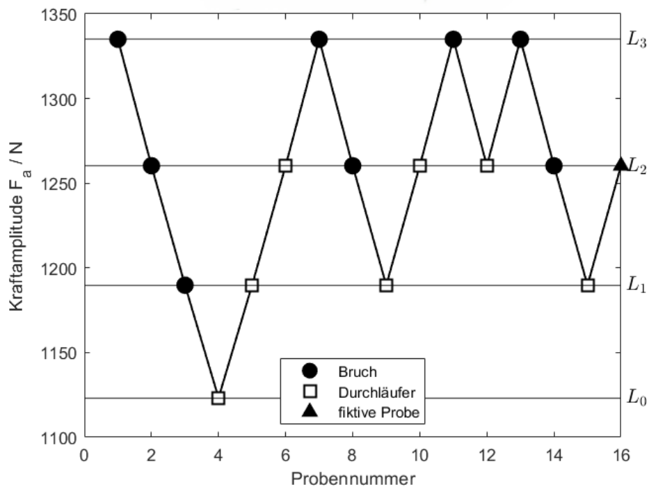
Abbildung 4.7.: Darstellung der ausgewerteten Treppenstufenfolge.
