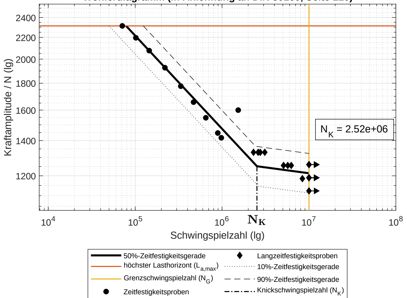
Wöhlerdiagramm (In Anlehnung an DIN 50100, Seite 110)
